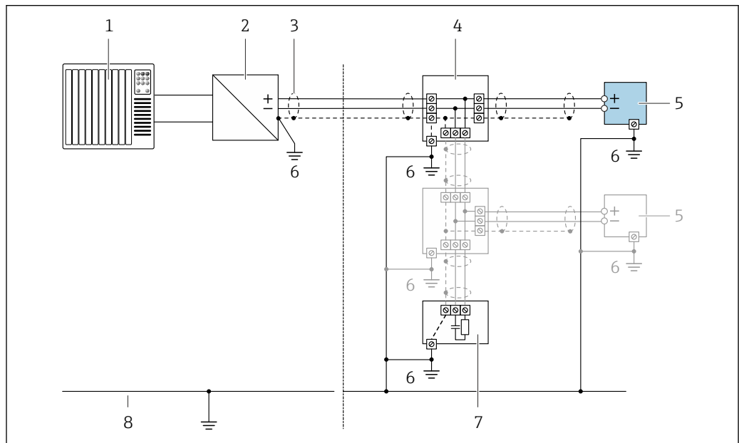
20 Esempio di connessione per FOUNDATION Fieldbus
