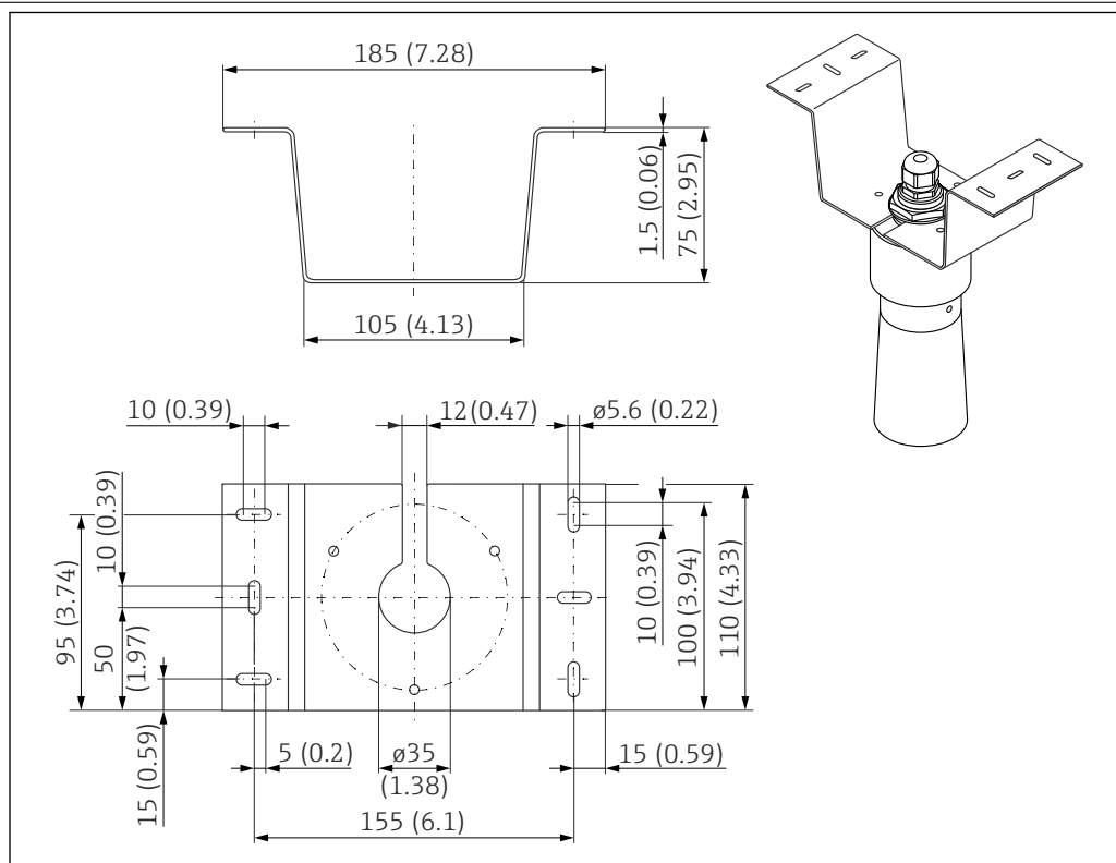
20 Monteringsbrakett for takmontering. Måleenhet mm (in)
