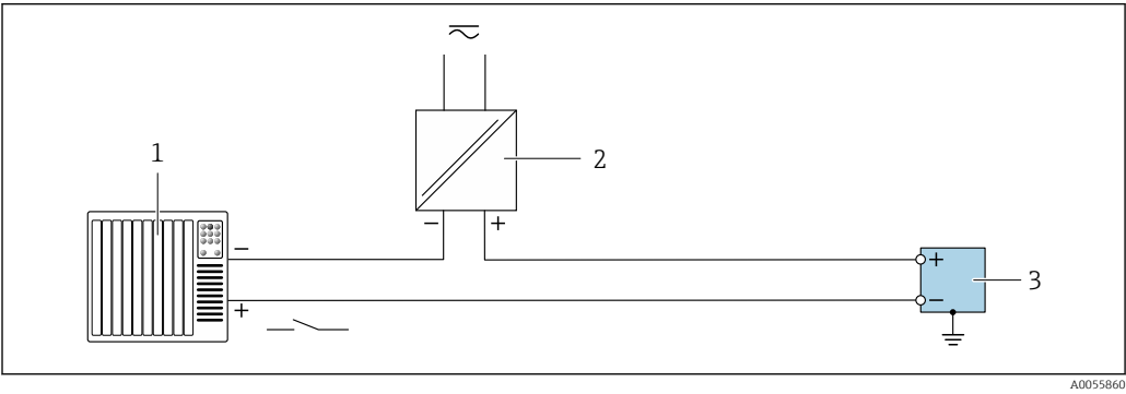
25 Ejemplo de conexión de una entrada de estado 1 Sistema de automatización con salida de conmutación pasiva (p. ej., PLC) 2 Alimentación 3 Transmisor con entrada de estado
