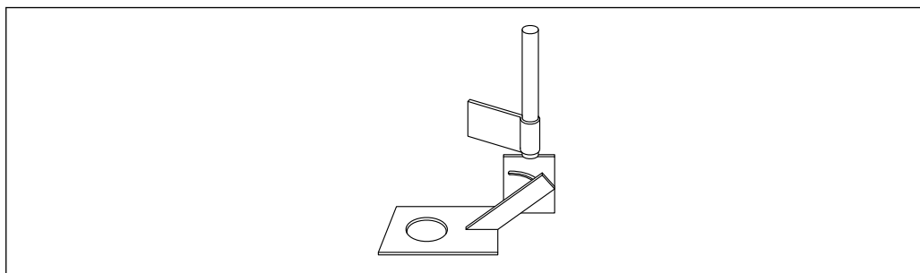
図 31 汎用ホルダ、1.4301、傾斜機構および固定ヘッド付き、センサ切り欠き \varnothing 108 mm (4.25 in)
