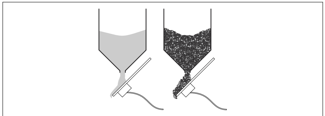
図 7 砂と砂利を測定するための丸型センサをサイロ排出ハッチの下に設置
