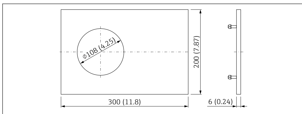
図 30 バッフルプレート、1.4301、センサ切り欠き \varnothing 108 mm (4.25 in)。測定単位 mm (in)
