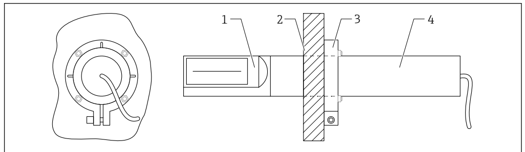
図 6 ロッドセンサの取付け（背面図）
