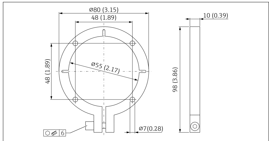
図 24 取付フランジ、1.4301、ロッドセンサ用
