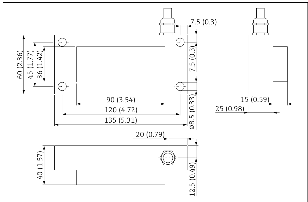
図 20 角型センサの寸法。測定単位 mm (in)
