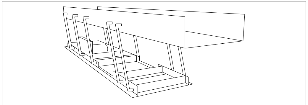
図 13 振動シュート
