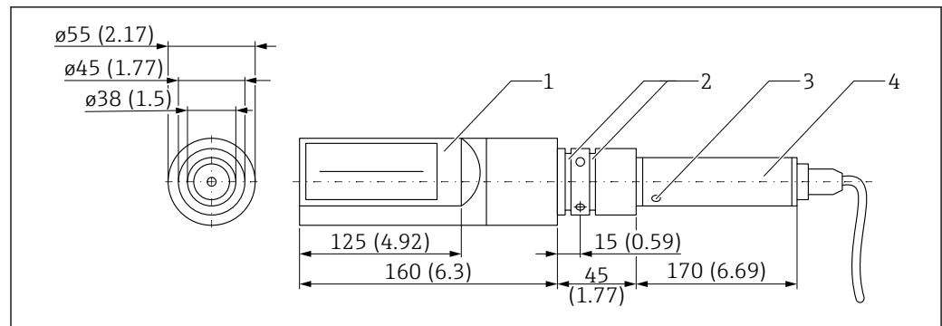
図 23 ロッドセンサの寸法。測定単位 mm (in)
