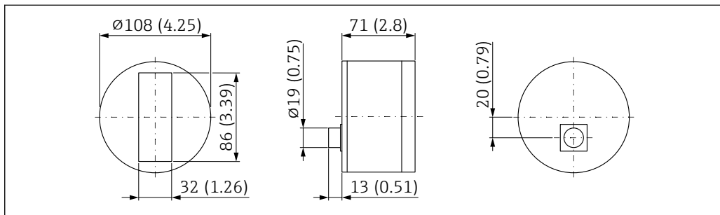
図 18 丸型センサ（ミドル）の寸法。測定単位 mm (in)
