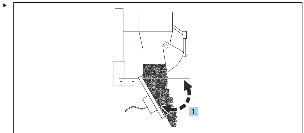
図 9 研磨性のある粉粒体：バッフルプレート / 開口部ハッチの位置
