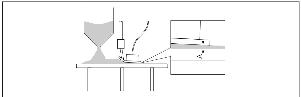
図 10 コンベヤーベルトの上への丸型センサの設置
