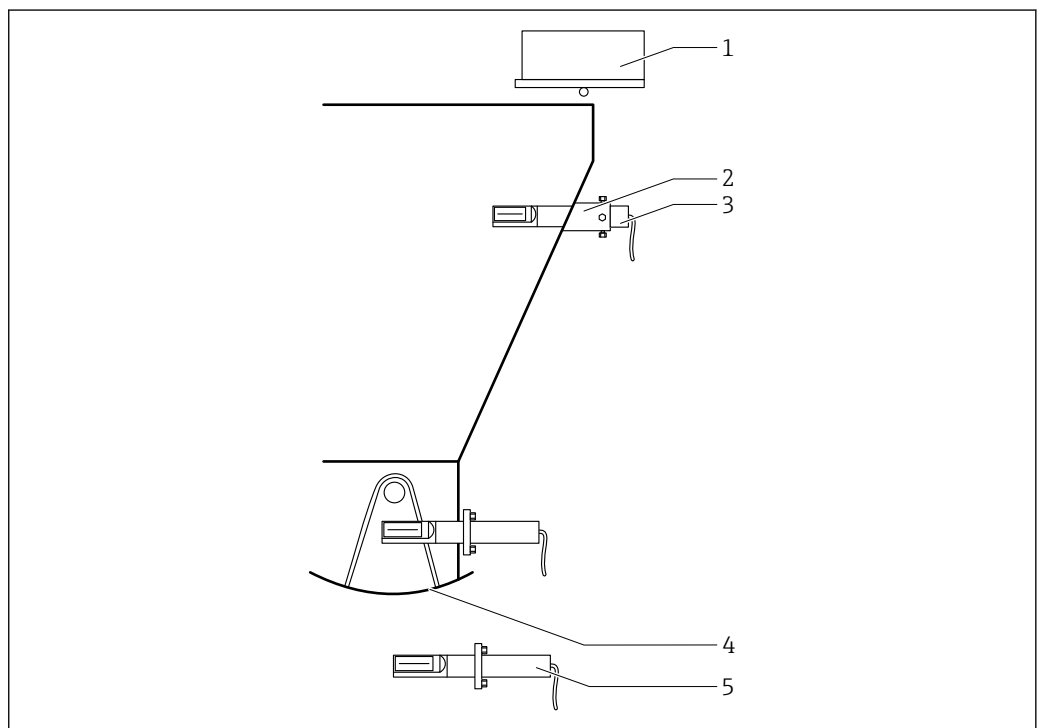
図 14 サイロへのロッドセンサの設置
