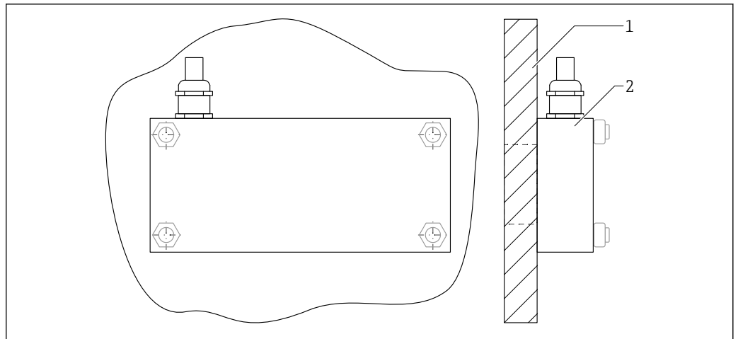
図 5 角型センサの取付け（背面図）
