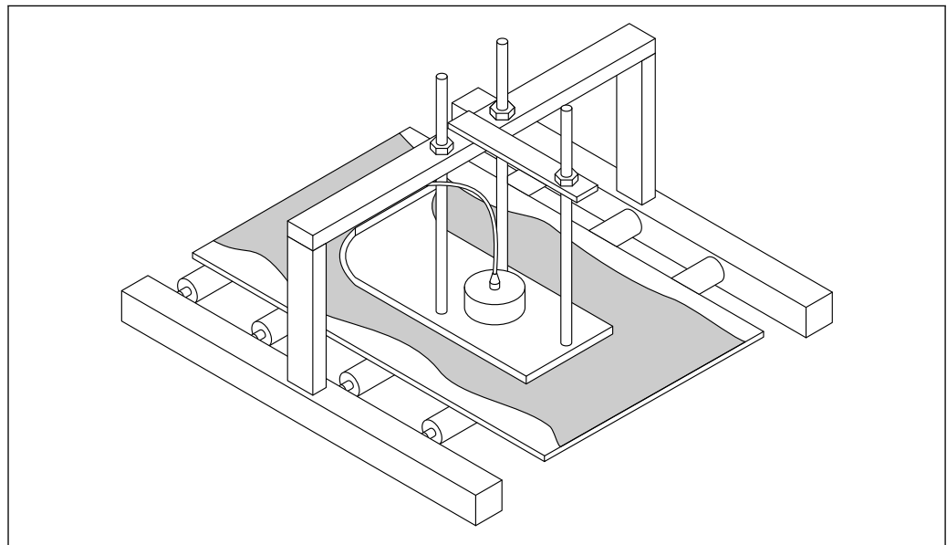
図 12 スライディングキャリッジの設置例
