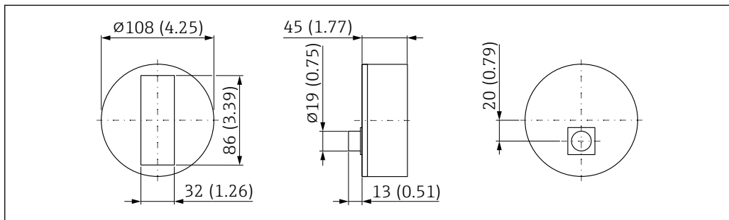
図 17 丸型センサ（ショート）の寸法。測定単位 mm (in)
