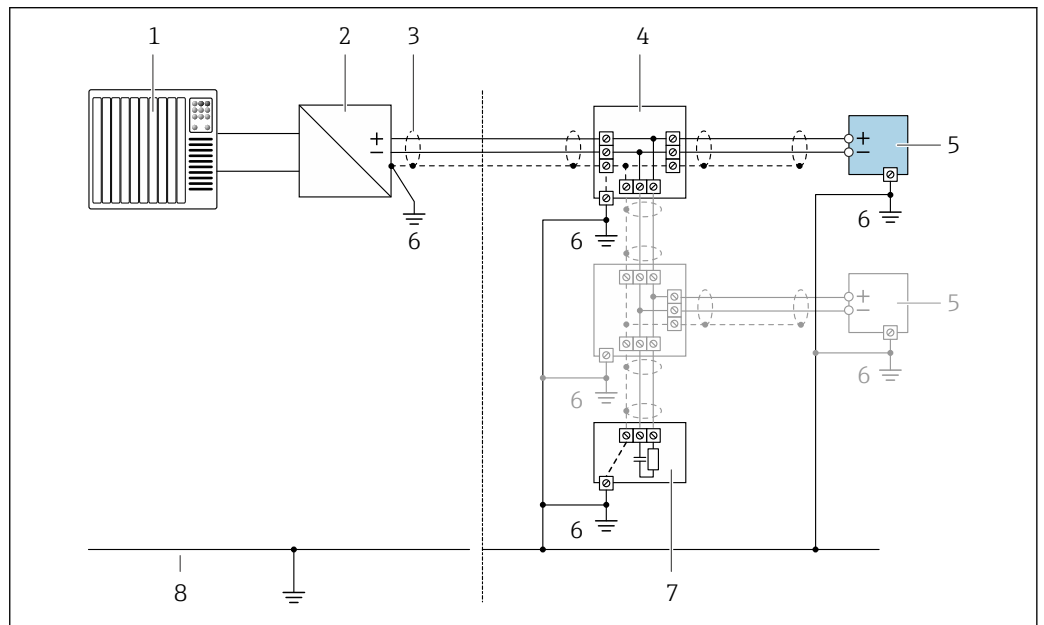
20 Ejemplo de conexión de FOUNDATION Fieldbus
