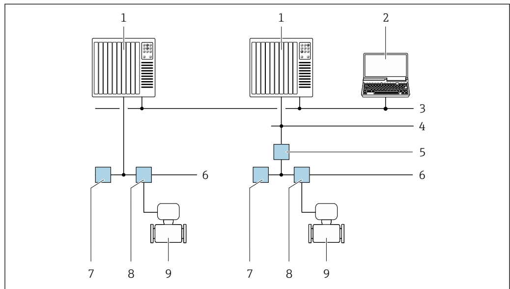
26 Opciones para la configuración a distancia mediante red FOUNDATION Fieldbus
