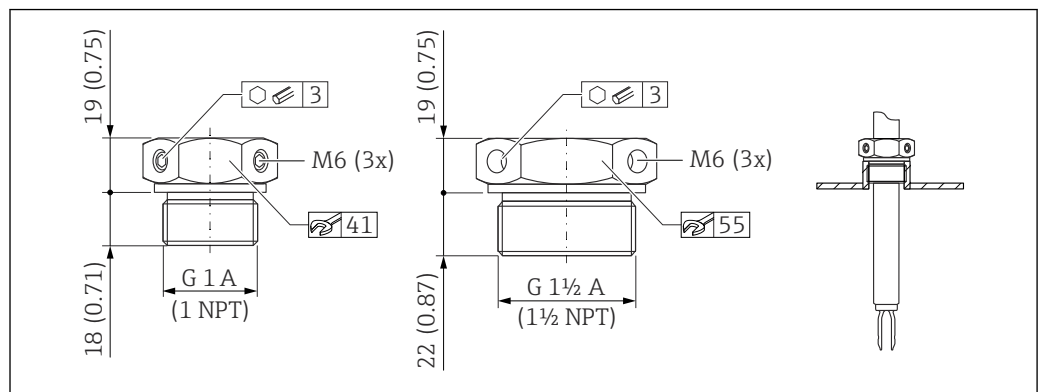
25 Manchons coulissants pour un fonctionnement sans pression p_e = 0 \text{ bar} (0 psi). Unité de mesure mm (in)
