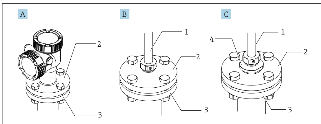
19 Bridas
