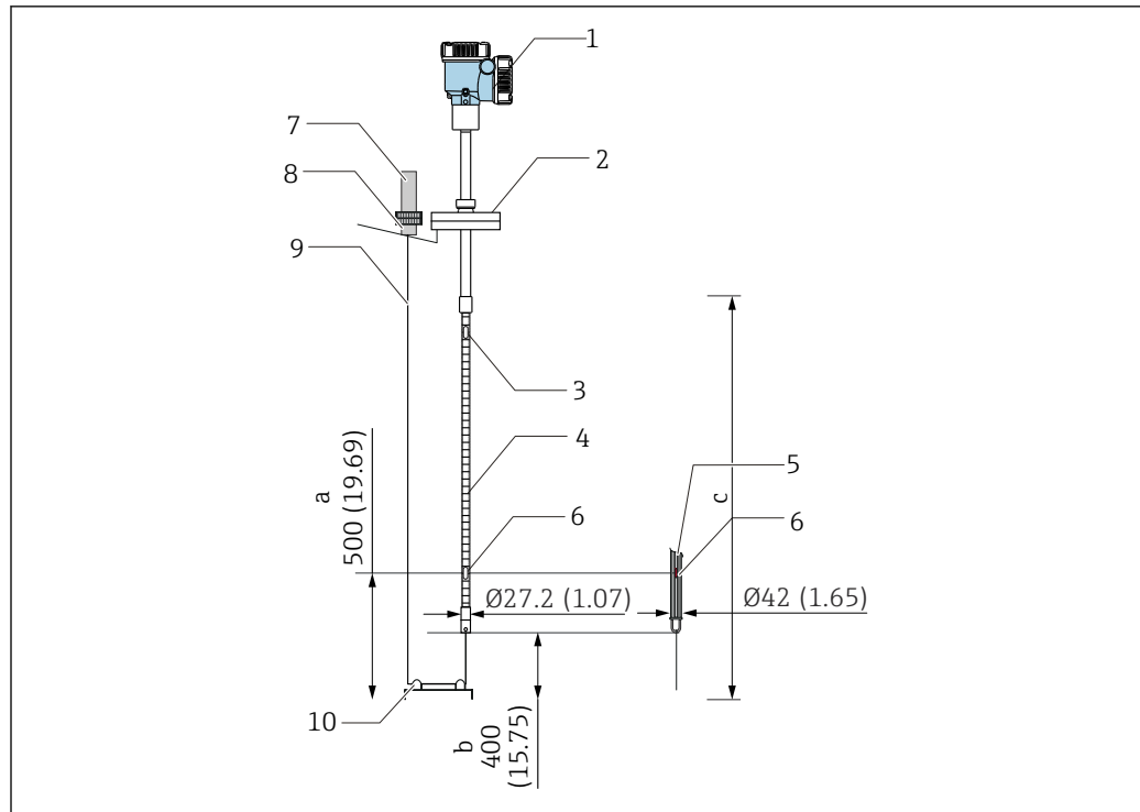
24 Método de anclaje superior. Unidad de medida mm (in)
