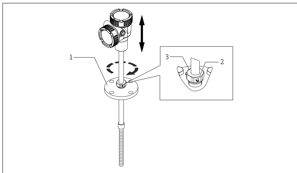
21 Tipo de ajuste de altura del NMT81
