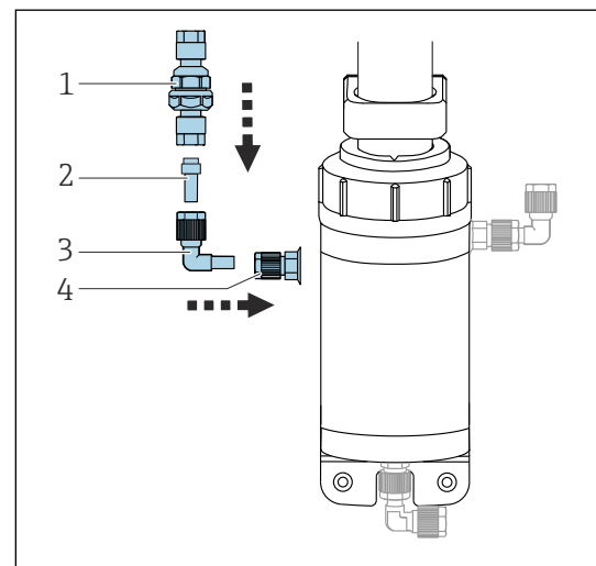
17 Montere rengjøringstilkoblingen 1 Sikkerhetsventil 2 Nippel 3 Vinkeltilkobling 4 Slangetilkobling
