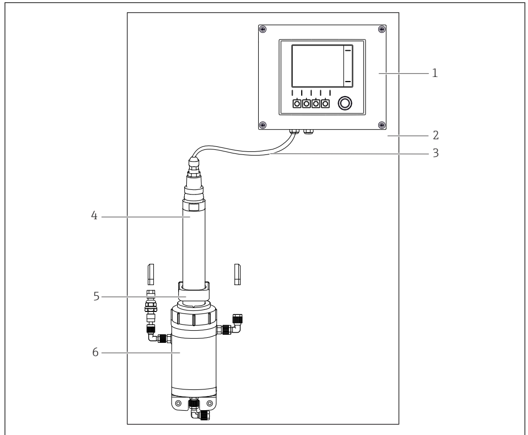
13 Målesystem
