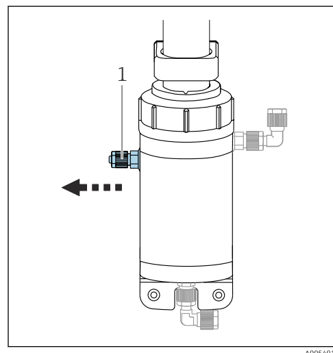
16 Klargjøre rengjøringstilkoblingen 1 Slangetilkobling med tetningsplugg
