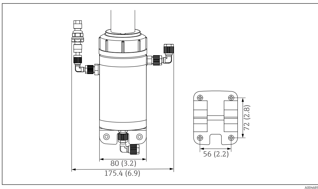
4 Mål på standardarmatur CFS51 med monteringsplate (høyre). Enhet: mm (in)
