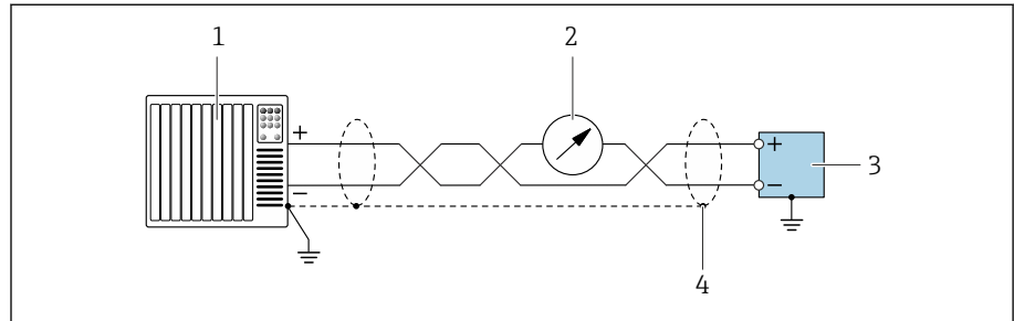
17 Exemple de raccordement pour sortie courant 4 ... 20 mA avec HART (active)
