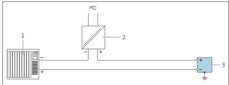
19 Exemple de raccordement pour sortie impulsion / sortie fréquence / sortie tout ou rien (passive)
