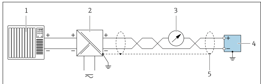
18 Exemple de raccordement pour sortie courant 4 ... 20 mA avec HART (passive)
