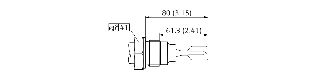
図 33 ネジ接続 ISO228 G 1。測定単位 mm (in)
