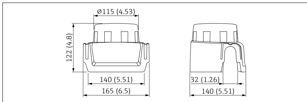
図 43 アルミニウム製シングルコンパートメントハウジング用保護カバー。測定単位 mm (in)
