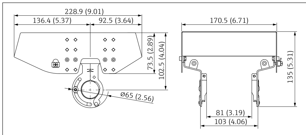
図 42 デュアルコンパートメントハウジング用の日除けカバー。測定単位 mm (in)
