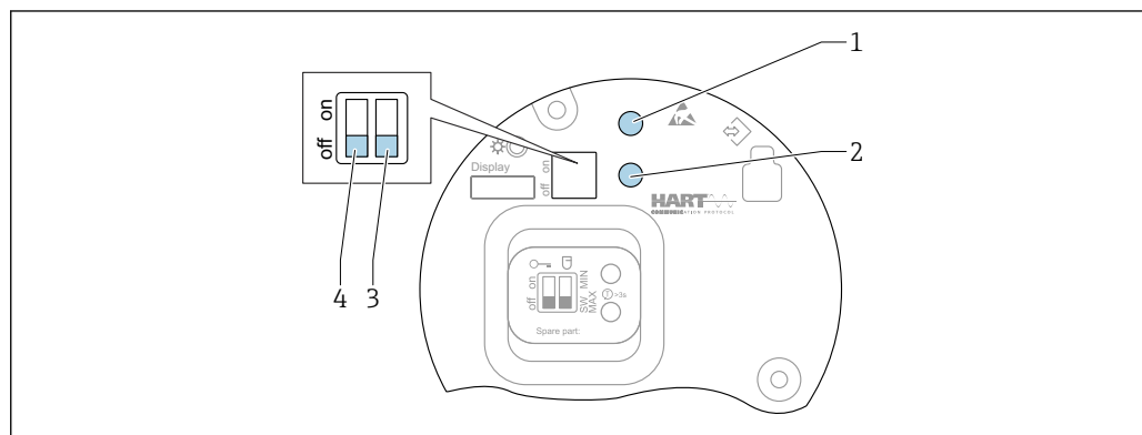
図 40 FEL60H エレクトロニックインサートの操作キーおよび DIP スイッチ
