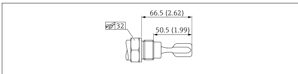
図 32 ネジ接続 ISO228 G 3/4。測定単位 mm (in)
