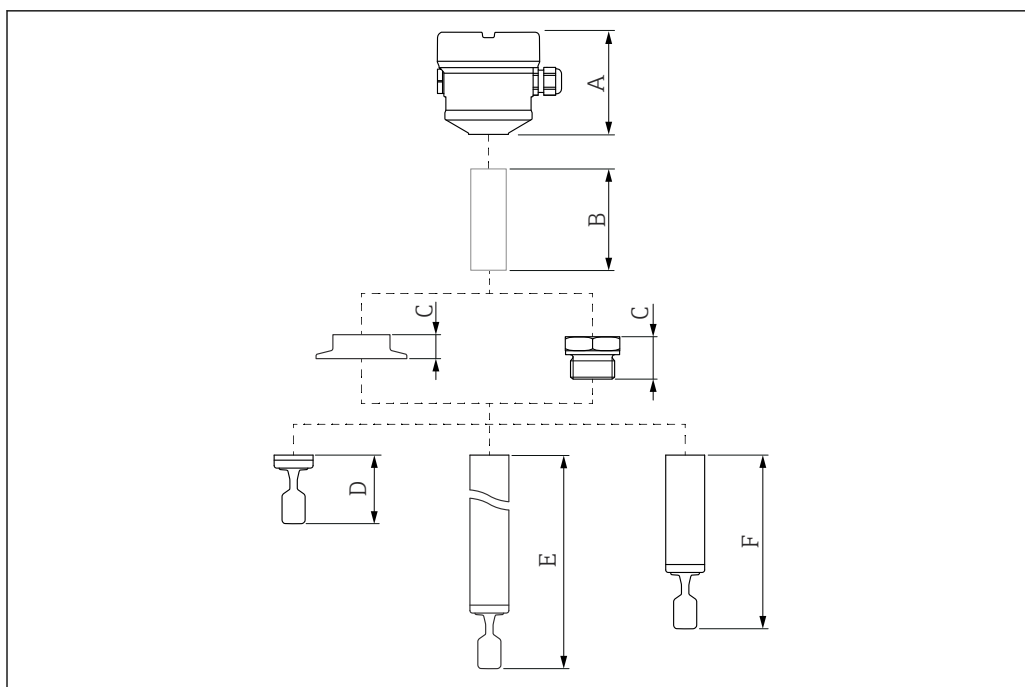
図 22 本体高さを計算するための構成品
