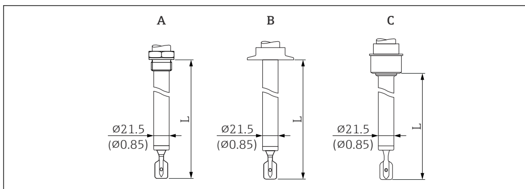
図 29 プローブ型式：伸長パイプ、ショートパイプ（センサ長 L）。測定単位 mm (in)
