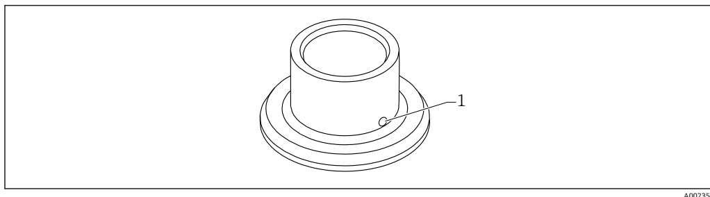
図 44 漏れ検知用の穴付きの溶接アダプタ (例)
