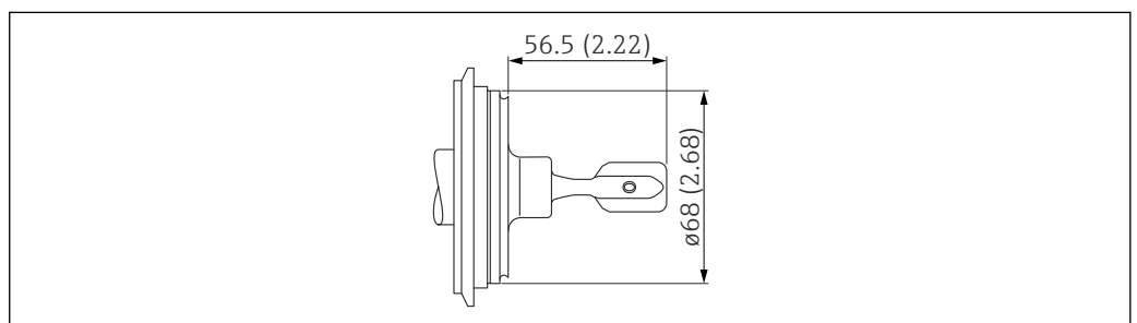
37 バリベント N パイプ DN65-162 PN25。測定単位 mm (in)
