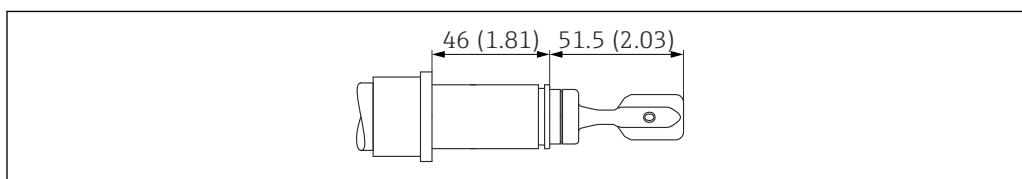
図 34 Ingold アダプタ 25 x 46 mm (2.52 in)。測定単位 mm (in)
