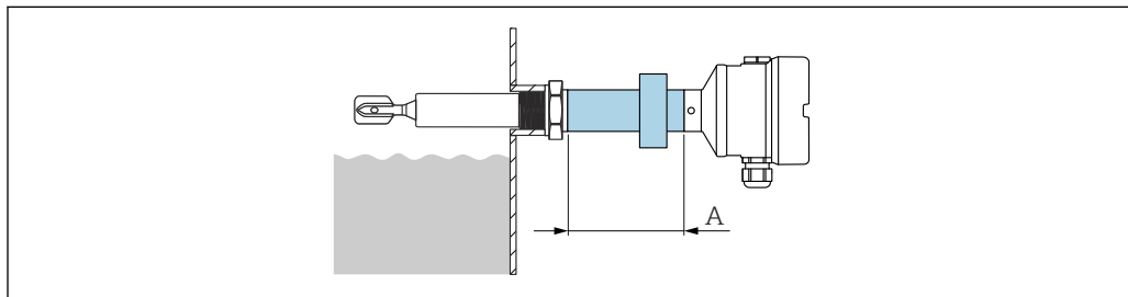
図 27 伸長パイプ用の耐圧防爆対応ガスタイトフィードスルー
