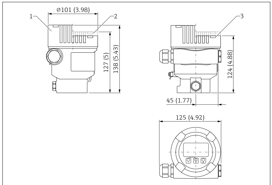
24 シングルコンパートメントハウジング、アルミニウム、コーティングの寸法。測定単位 mm (in)
