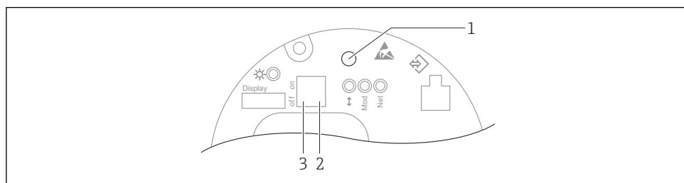
20 Tecla de configuración y microinterruptores en el módulo del sistema electrónico (FEL60P), Ethernet-APL
