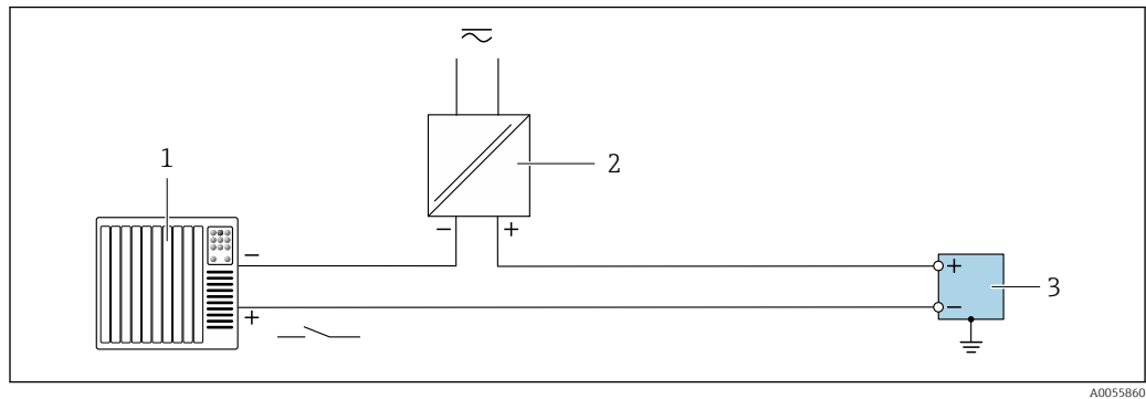
19 Anschlussbeispiel für Statuseingang
