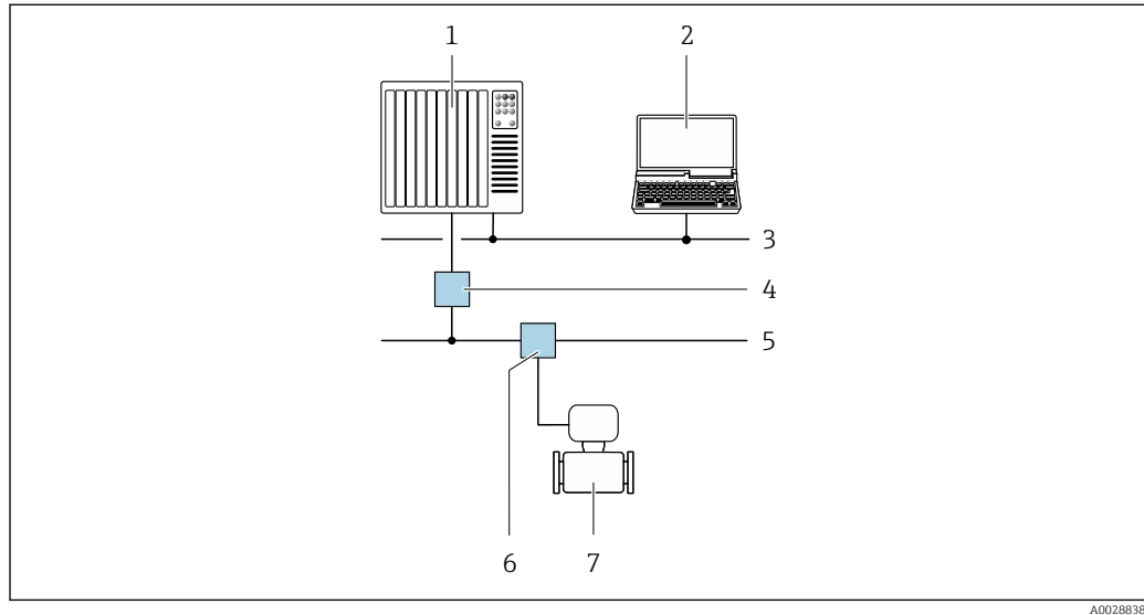
25 Möglichkeiten der Fernbedienung via PROFIBUS PA Netzwerk
