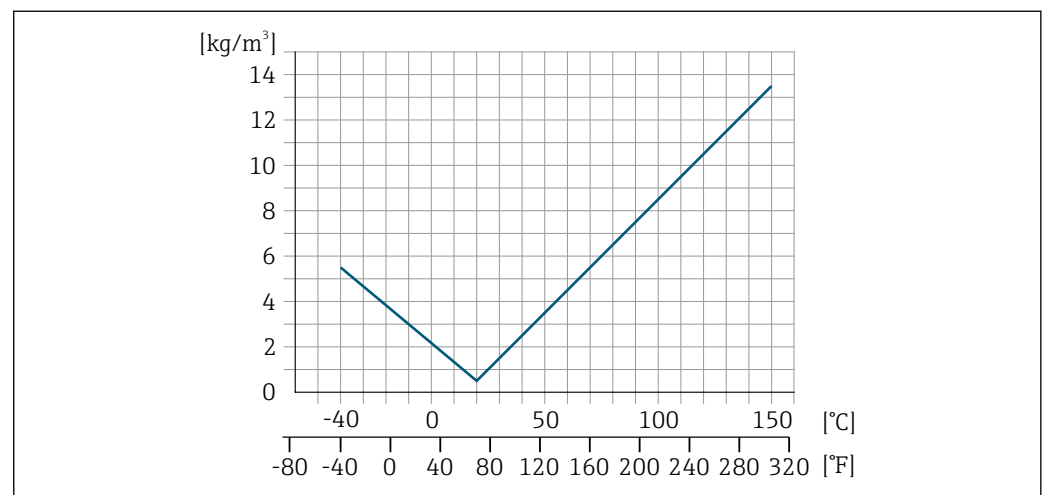
35 Felddichtejustierung, Beispiel bei +20 \text{ }^\circ\text{C} ( +68 \text{ }^\circ\text{F} )
