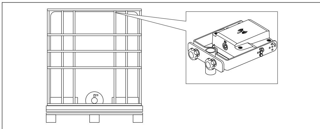
3 Установка с помощью монтажного кронштейна для трубок еврокуба
