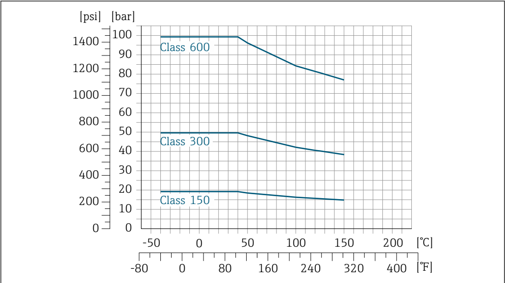
24 Con material de la brida 1.4404 (F316/F316L)
