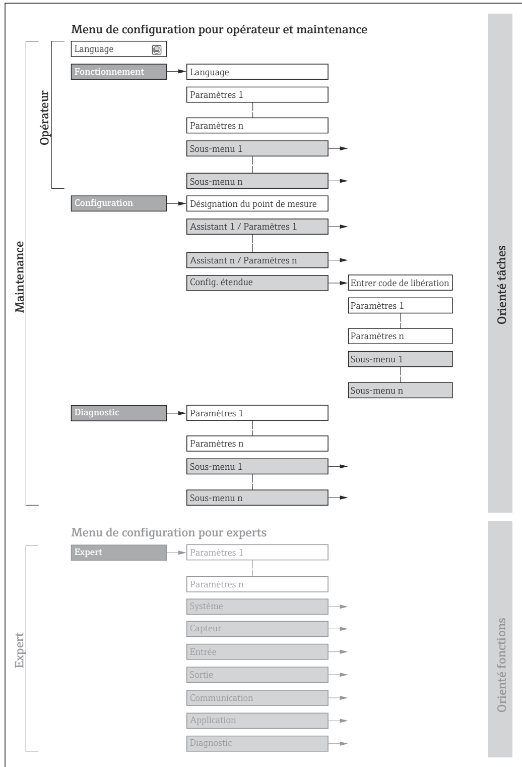
11 Structure schématique du menu de configuration
