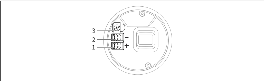
图 5 接线腔中的接线端子和接地端
