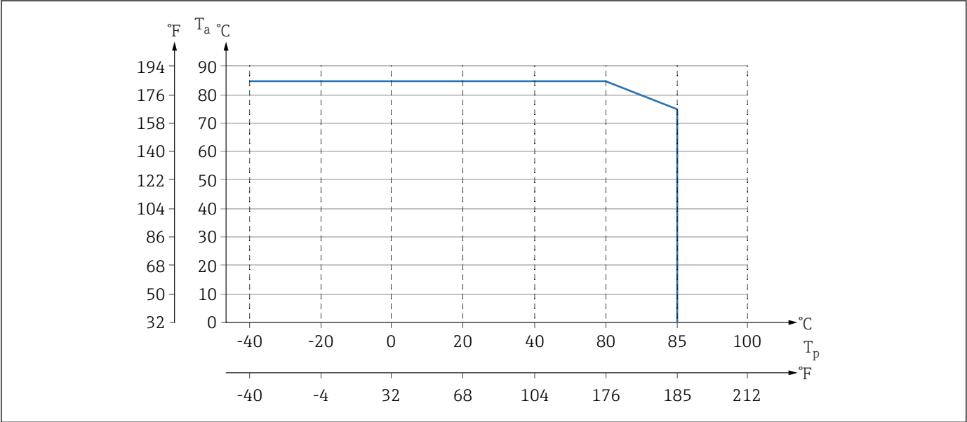
图 13 以上为无保温层竖直安装时的温度范围。
