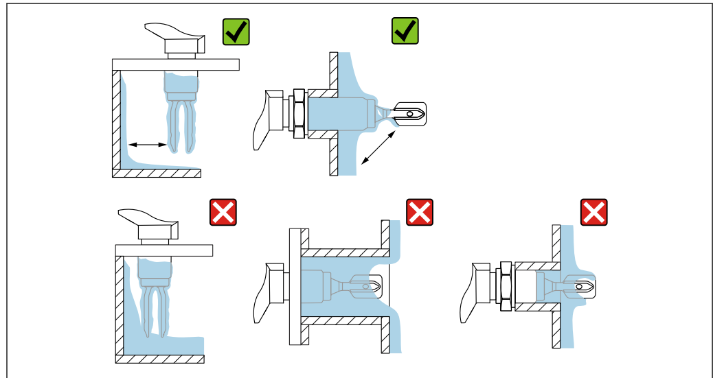
10 Ejemplos de instalación para un producto de proceso altamente viscoso
