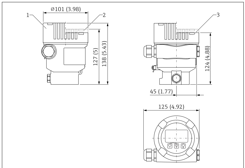
24 Medidas de la caja de compartimento único, aluminio, recubierta. Unidad de medida mm (in)
