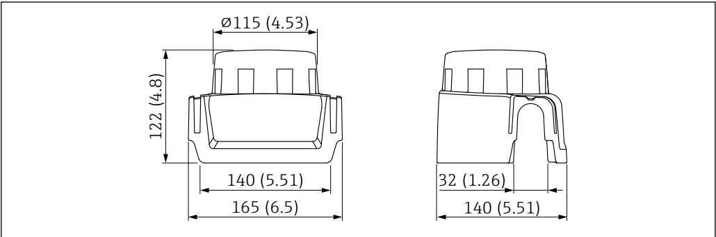
47 Cubierta protectora para caja de compartimento único de aluminio. Unidad de medida mm (in)
