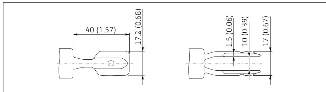
31 Horquilla vibrante. Unidad de medida mm (in)
