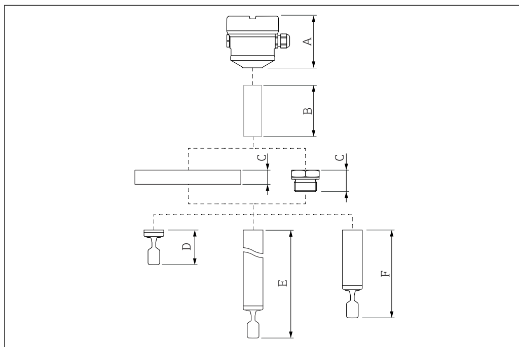
22 Componentes para determinar la altura del equipo
