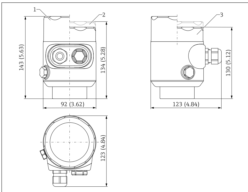
25 Medidas de la caja de compartimento único, 316L, higiénica. Unidad de medida mm (in)
