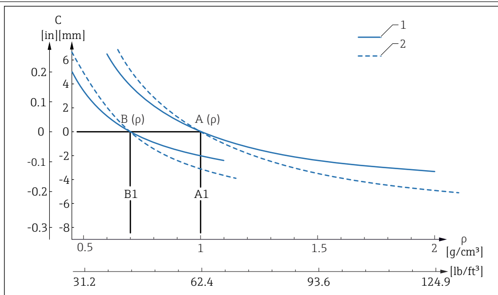
6 Desviación del punto de conmutación sobre la densidad
