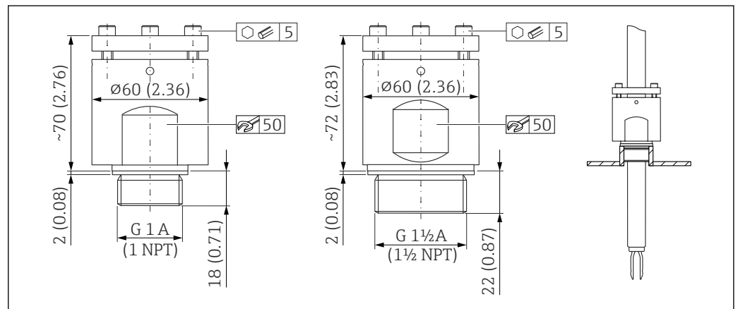
50 Casquillos deslizantes para alta presión. Unidad de medida mm (in)
