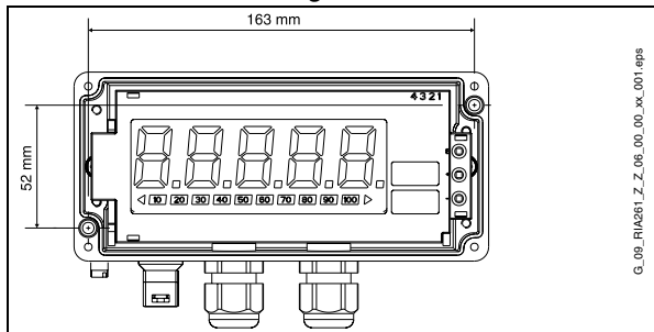
Abb. 2: Direkte Wandmontage
