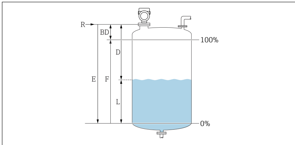
16 Konfigurationsparameter för nivåmätning hos vätskor
