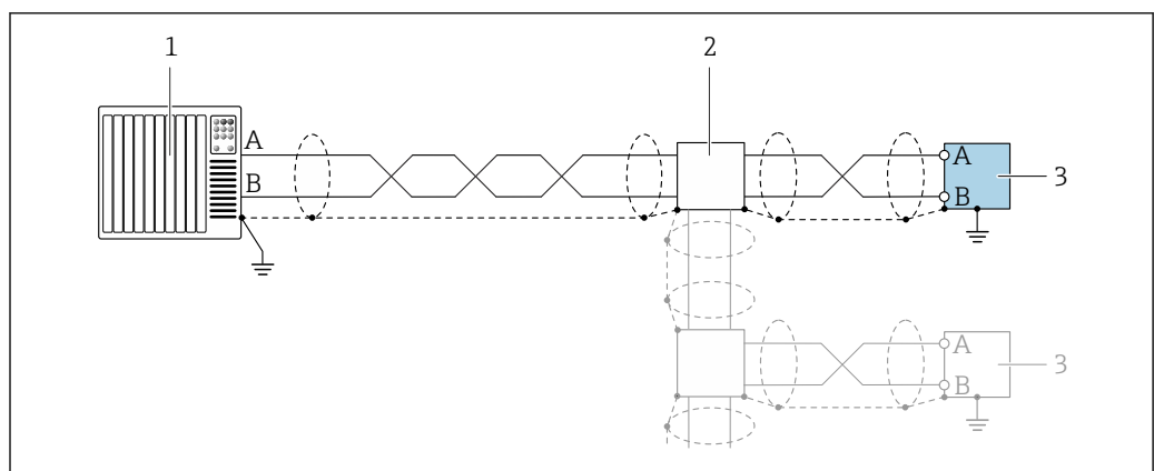
16 Exemple de raccordement pour Modbus RS485
