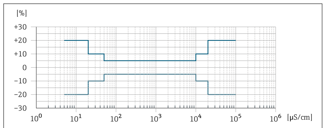
33 Écart de mesure (en option : caractéristique de commande "Mesure de conductivité étalonnée", option CW)
