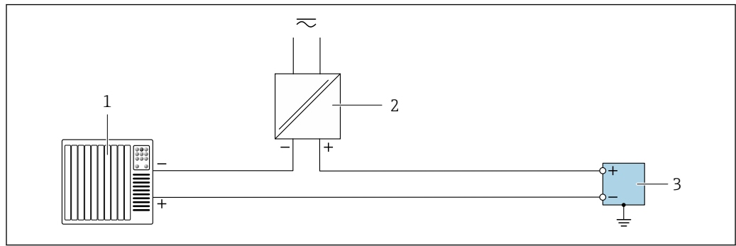
14 Exemple de raccordement pour sortie relais
