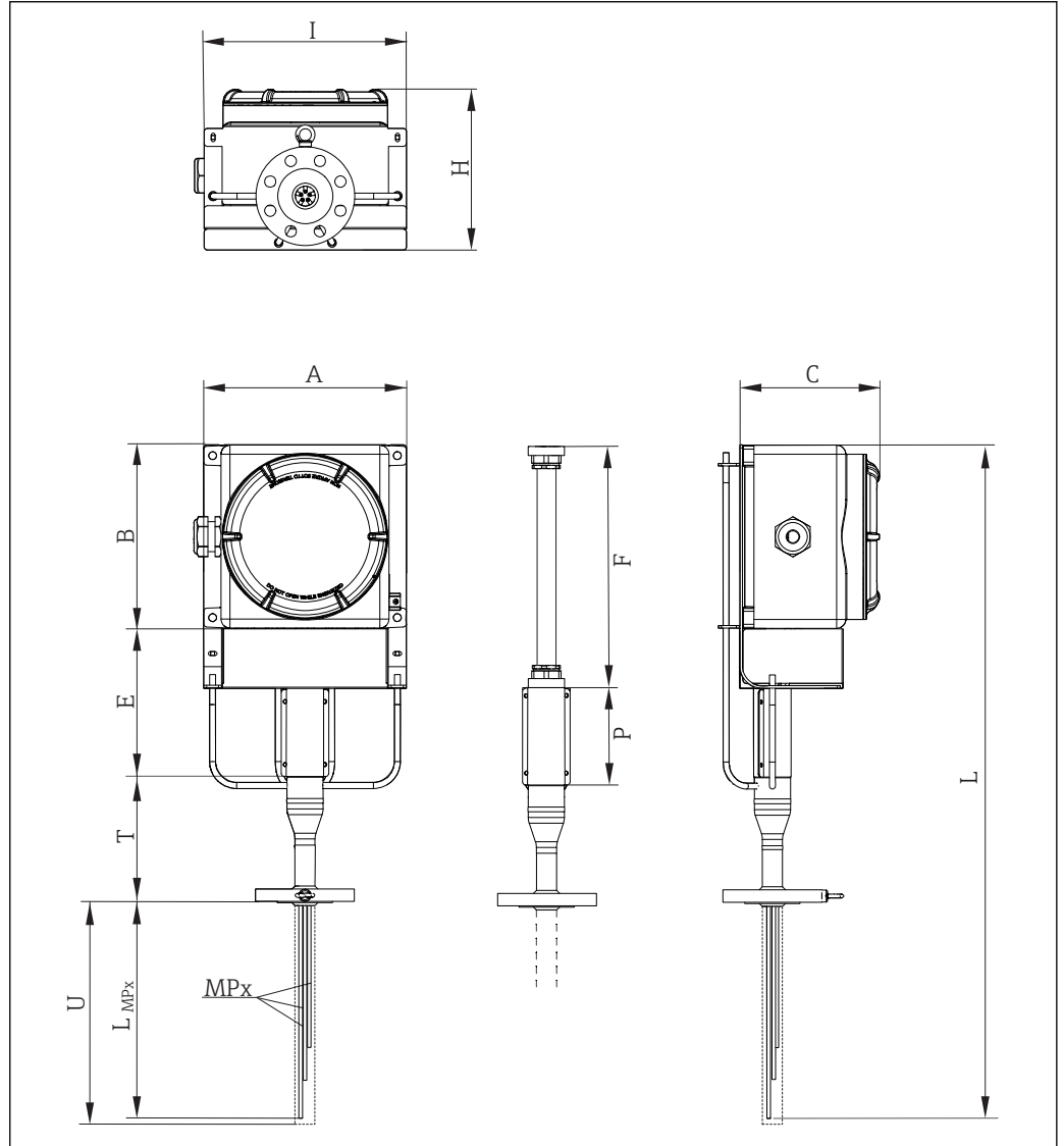
4 Construction du capteur de température multipoint modulaire, avec extension du châssis. Toutes les dimensions en mm (in)
