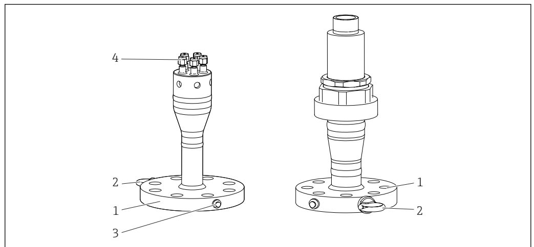
6 Bride en tant que raccord process
