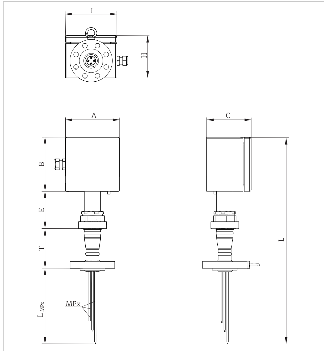
5 Construction du capteur de température multipoint modulaire, avec tube prolongateur. Toutes les dimensions en mm (in)
