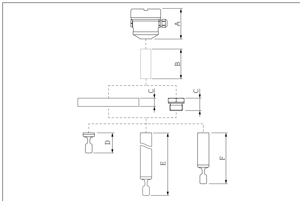
13 Компоненты, по которым определяется высота прибора
