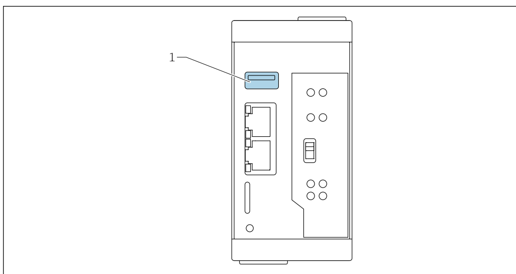
39 Расположение USB-порта
