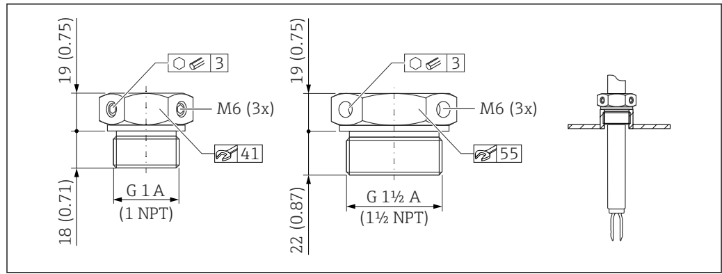
42 Скользящие муфты для использования при отсутствии избыточного давления, p_e = 0 бар (0 фунт/кв. дюйм). Единица измерения мм (дюйм)
