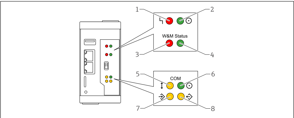
36 Описание состояний светодиодов
