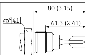
24 Резьба ISO 228 G 1. Единица измерения мм (дюйм)
