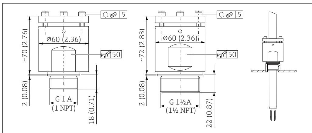
43 Скользящие муфты для использования в условиях высокого давления. Единица измерения мм (дюйм)
