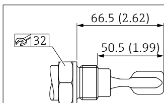
23 Резьба ISO 228 G 3/4. Единица измерения мм (дюйм)
