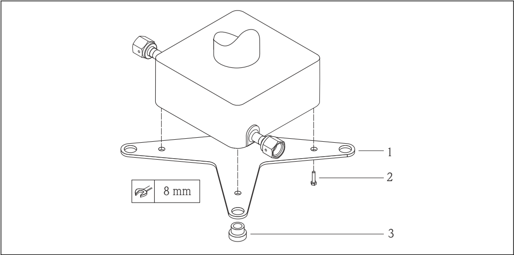
14 Kit di montaggio per piastra di montaggio per Cubemass
