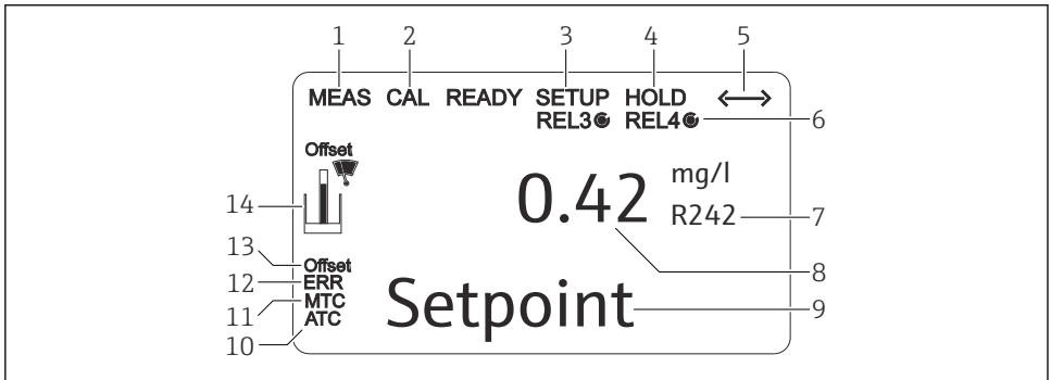
15 트랜스미터 LC 디스플레이
