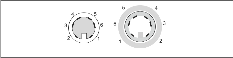
10 TOP68 연결부; 커넥터와 커플링의 핀 배열(접점 쪽에서 본 모습)
