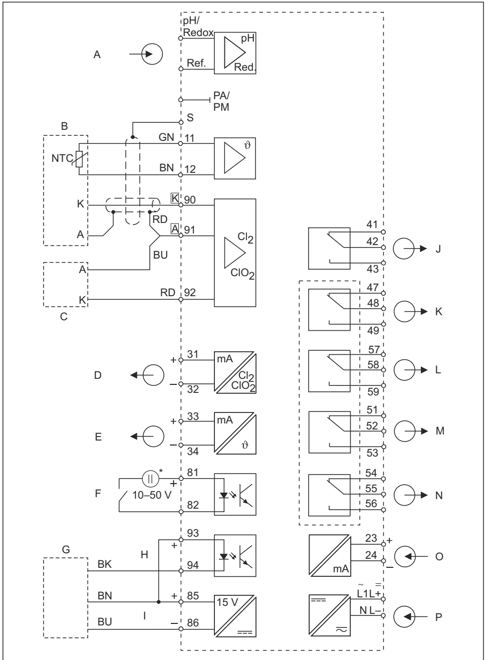
7 트랜스미터 전기 연결(버전 1)
