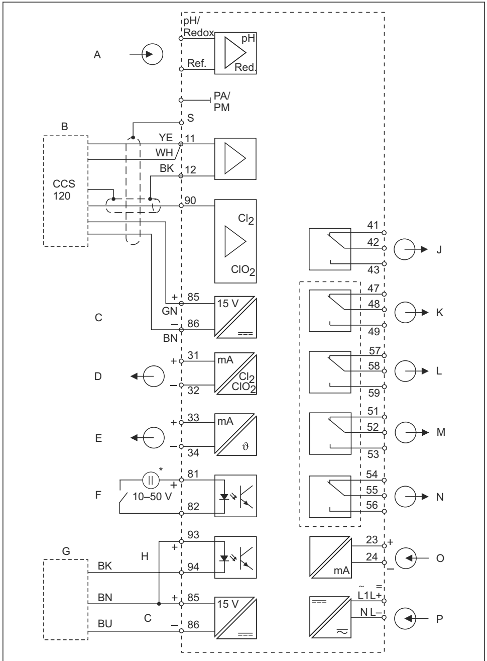
8 트랜스미터 전기 연결(버전 2)
