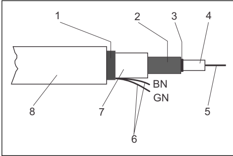
12 케이블 CMK 구조
