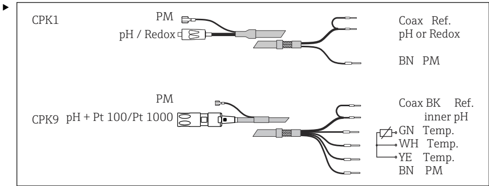
11 CPK1 또는 CPK9 케이블을 사용한 pH/ORP 센서 연결
