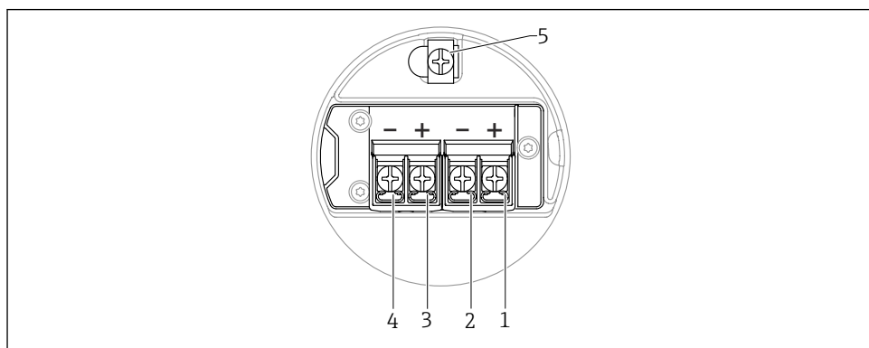
11 Asignación de terminales en el compartimento de conexiones; 4 ... 20 mA HART, salida de conmutación, caja de compartimento doble
