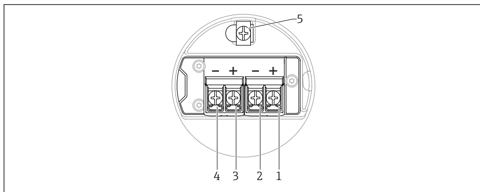
10 Asignación de terminales en el compartimento de conexiones; 4 ... 20 mA HART + 4 ... 20 mA analógico; caja de compartimento doble
