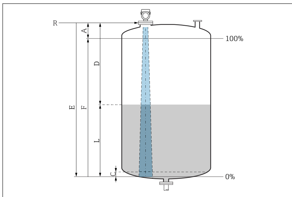
19 Parámetros de configuración para la medición de nivel en líquidos
