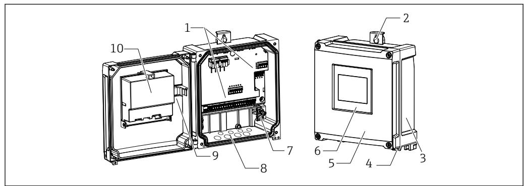
1 Estructura de la caja de policarbonato para montaje en campo
