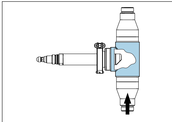
15 Installazione con armatura a deflusso CUA252
