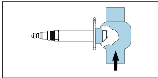
18 Installazione con connessione Varivent e corpo esteso
