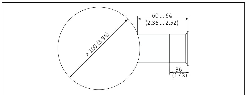
19 Connessione al tubo con adattatore a saldare. Dimensioni: mm (in)
