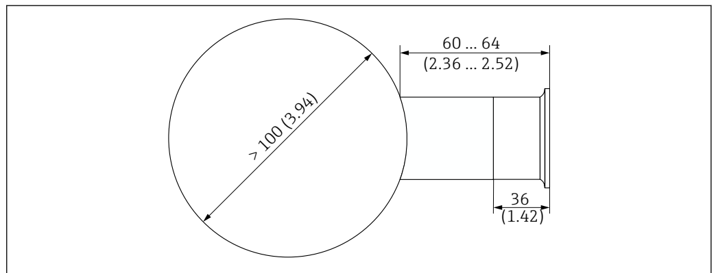
26 Connessione al tubo con adattatore a saldare. Unità: mm (in)
