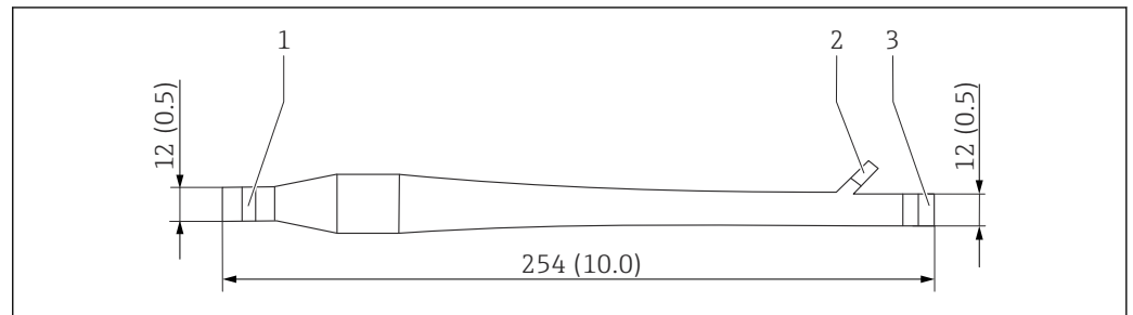
29 Degassatore. Unità: mm (in)
