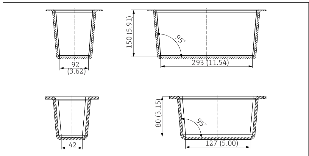
6 Recipiente di taratura grande (in alto) e recipiente di taratura piccolo (in basso). Unità ingegneristica: mm (in)
