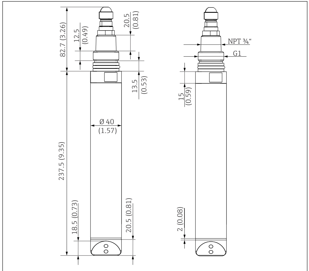
20 Dimensioni del sensore in plastica. Dimensioni: mm (in)
