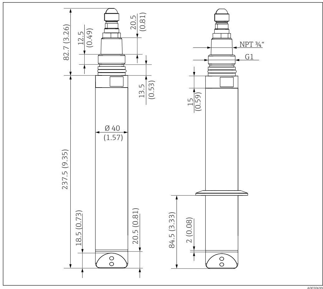
21 Dimensioni del sensore in acciaio inox e del sensore in acciaio inox con connessione clamp (a destra). Dimensioni: mm (in)
