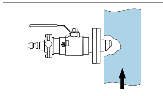
12 Installazione con armatura retrattile CUA451
