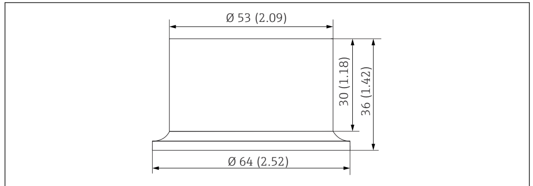
25 Adattatore a saldare. Unità: mm (in)
