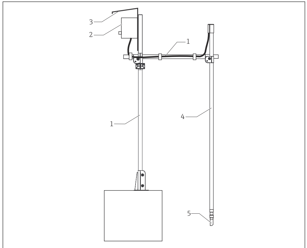
3 Esempio di sistema di misura con armatura ad immersione
