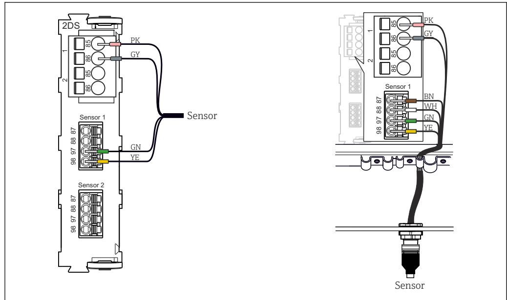
7 Collegamento del sensore sull'ingresso sensore (a sinistra) o mediante il connettore M12 (a destra)
