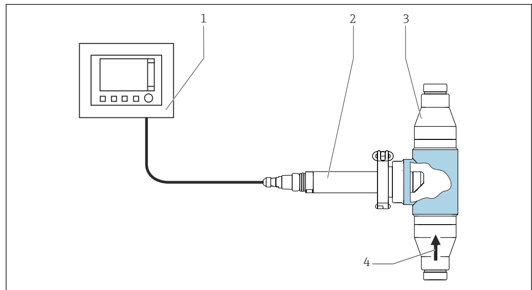
2 Esempio di sistema di misura con armatura a deflusso CUA252 per sensore in acciaio inox
