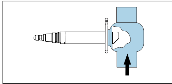
17 Installazione con connessione Varivent standard
