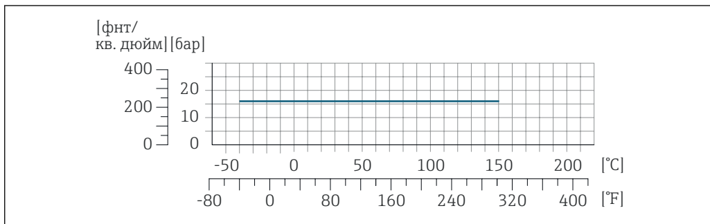
15 С материалом присоединения 1.4404 (316/316L)
