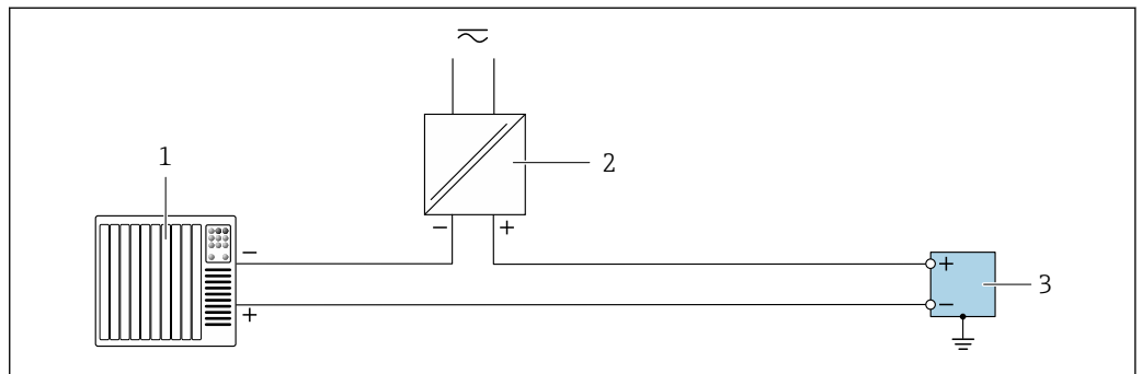
2 Пример подключения для импульсного/частотного/релейного выхода (пассивного)
