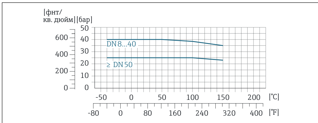
13 С материалом присоединения 1.4404 (316/316L)
