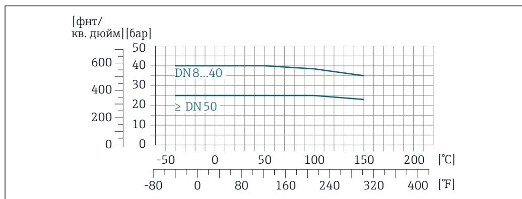
12 С материалом присоединения 1.4404 (316/316L)
