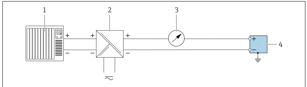
1 Пример подключения для токового выхода 4 до 20 мА (пассивного)
