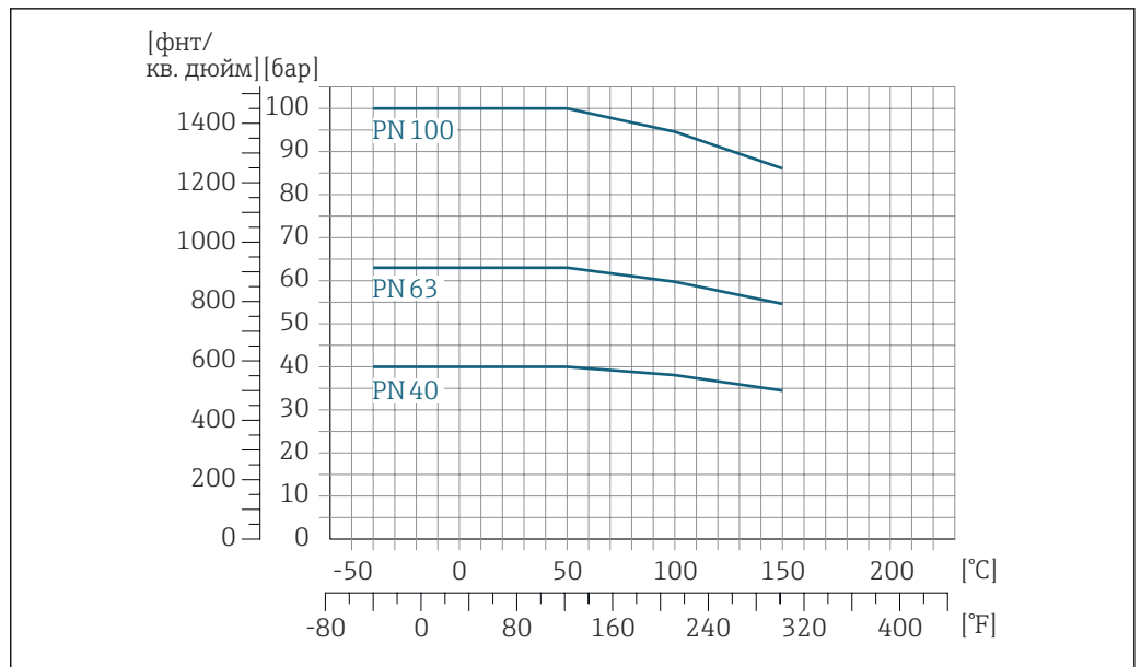
8 С материалом фланца 1.4404 (F316/F316L)
