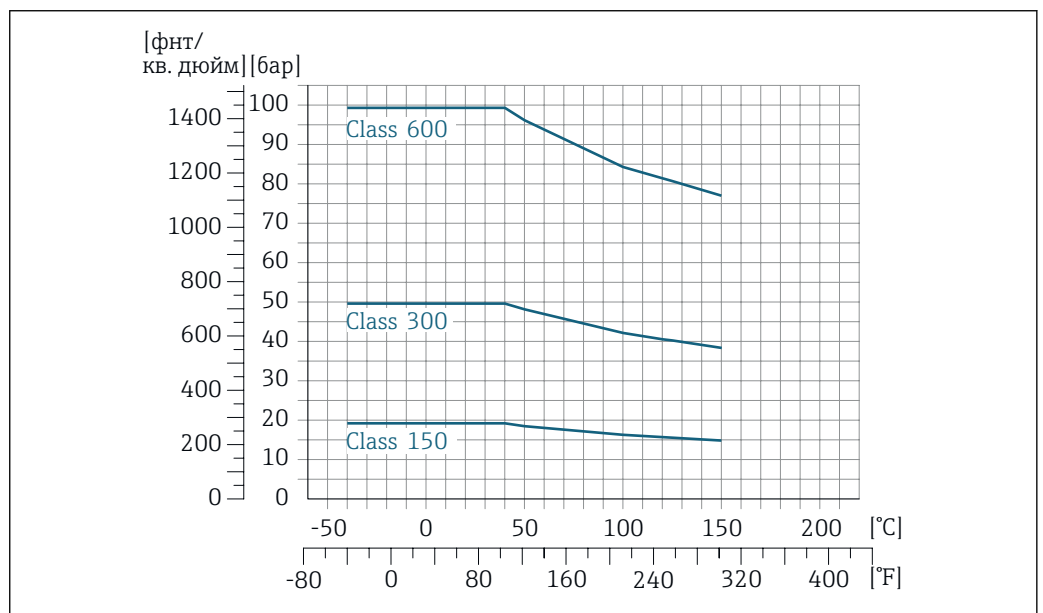
9 С материалом фланца 1.4404 (F316/F316L)
