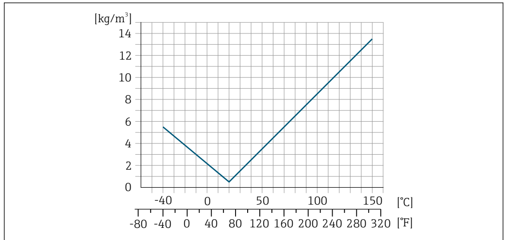
5 Калибровка по плотности на месте эксплуатации, в примере при +20 °C (+68 °F)
