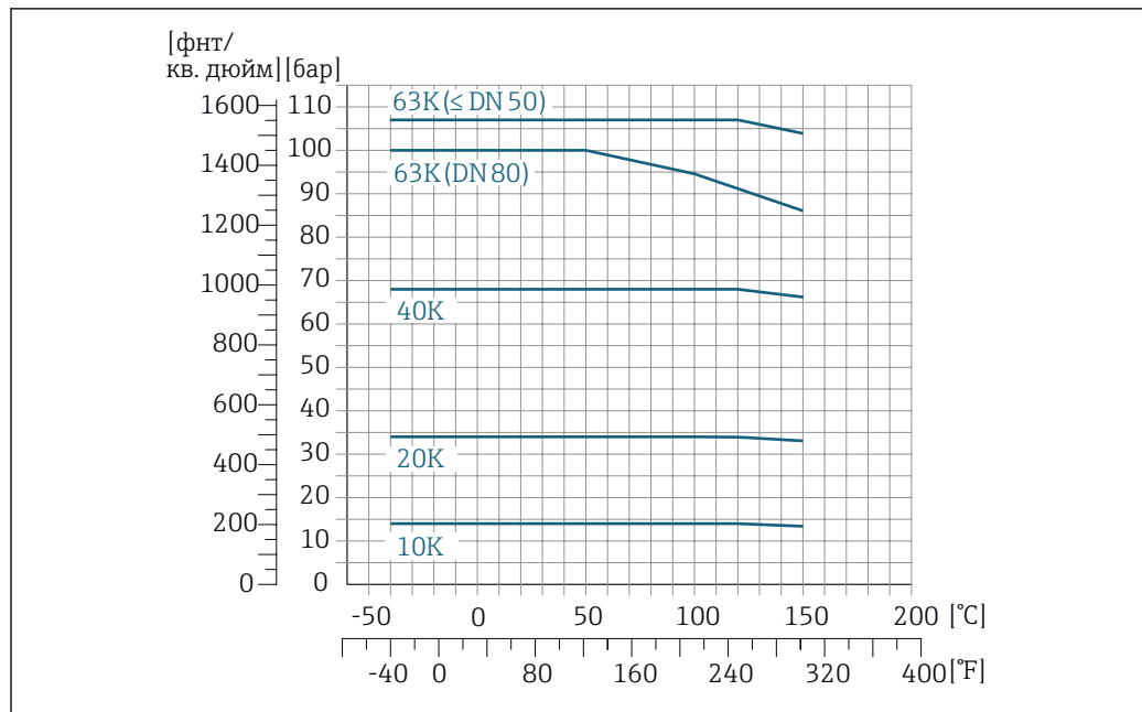
10 С материалом фланца 1.4404 (F316/F316L)
