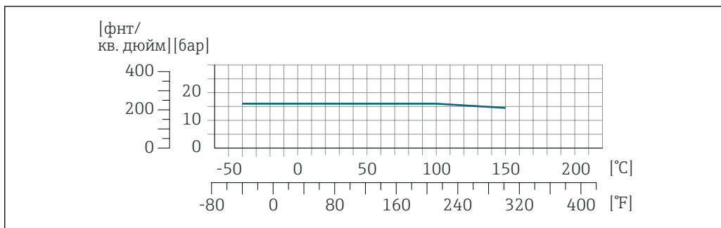
14 С материалом присоединения 1.4404 (316/316L)
