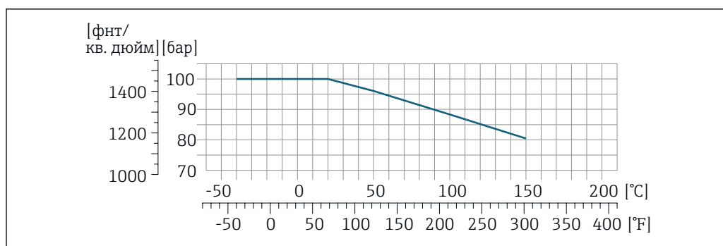
16 С материалом присоединения 1.4404 (316/316L)
