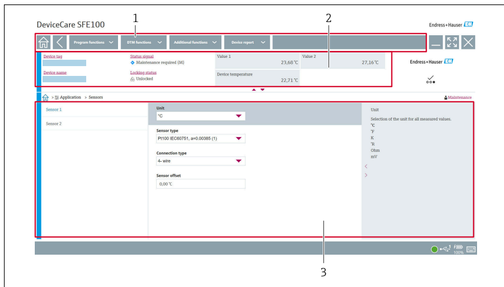
図 6 DeviceCare ユーザーインターフェースと機器情報
