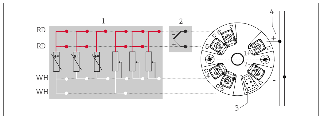
図 1 ヘッド組込型伝送器の端子接続の割当て
