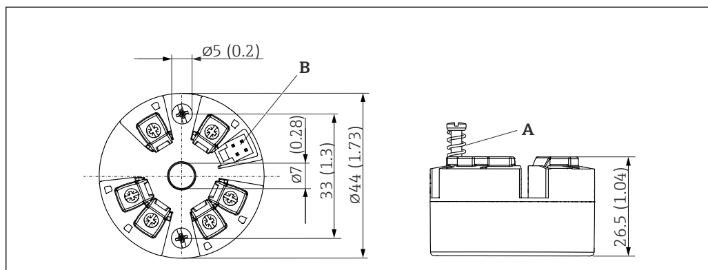
図 8 ネジ端子付きバージョン
