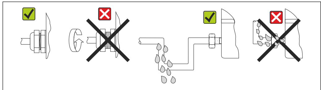
図 4 IP67 保護を維持するための接続のヒント
