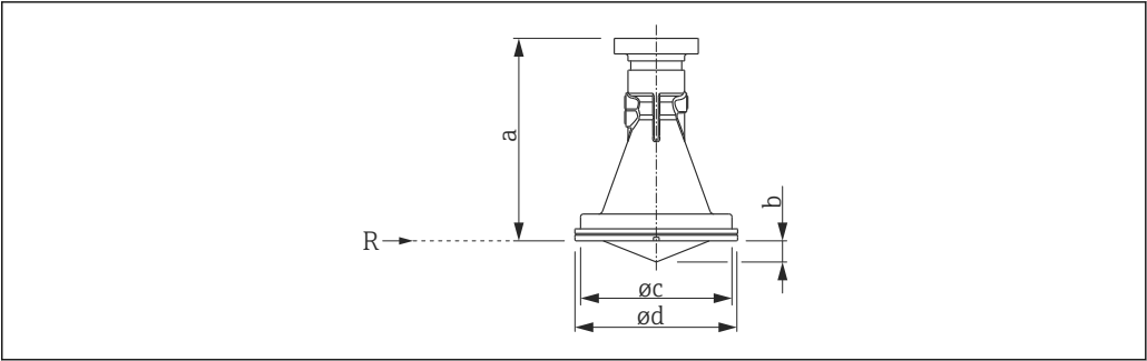
29 Dimensões do FMR56 sem conexão de processo. Unidade de medida mm (in)
