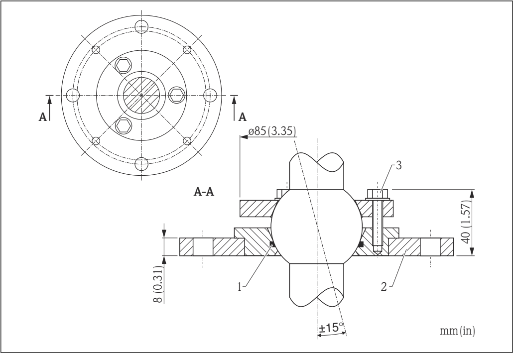
Unidade de alinhamento com flange UNI para FMR57
