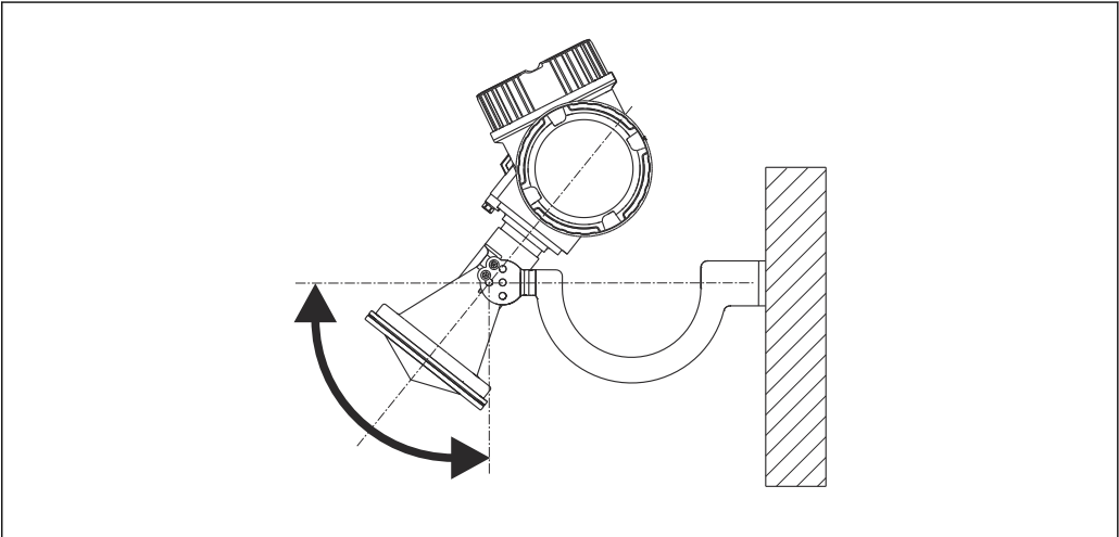
21 Instalação da antena piramidal com suporte de montagem
