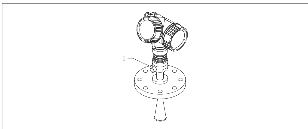
25 Micropilot FMR57 com conexão de purga de ar
