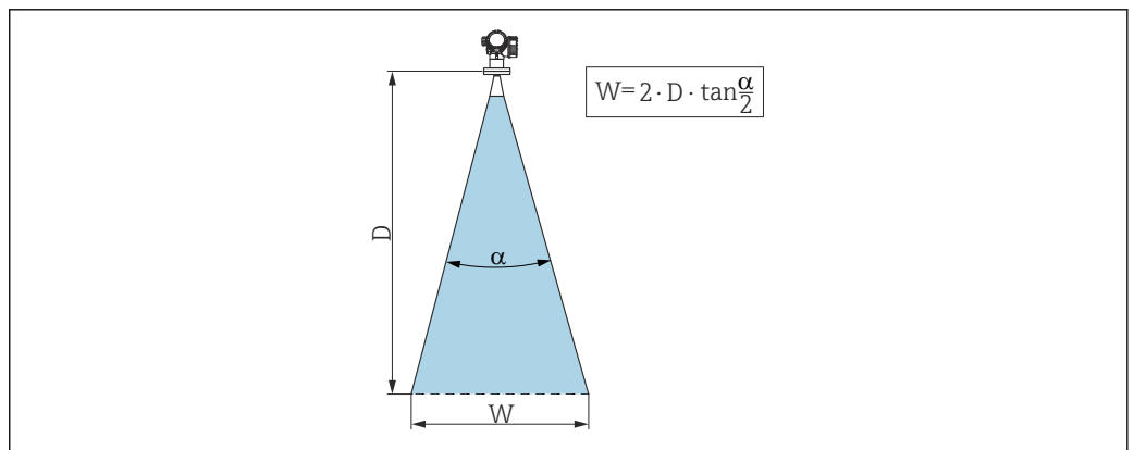
19 Relação entre o ângulo do feixe \alpha , a distância D e a largura do feixe W
