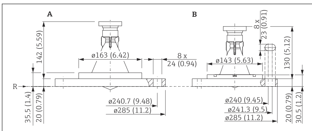
33 Dimensões do FMR56 com flange deslizante 6"/DN150. Unidade de medida mm (in)
