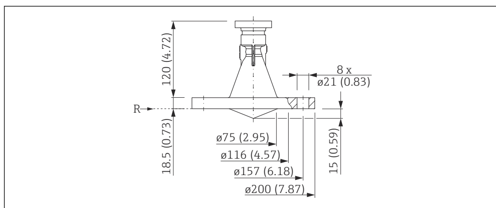
31 Dimensões do FMR56 com flange deslizante 3"/DN80. Unidade de medida mm (in)
