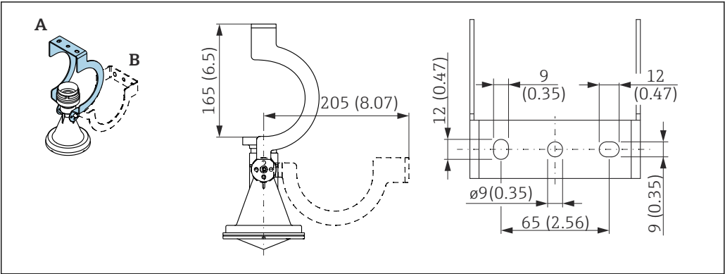
30 Dimensões do suporte de montagem. Unidade de medida mm (in)
