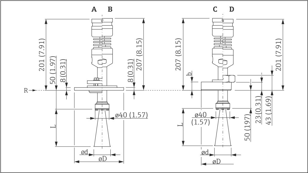
35 Dimensões do FMR57 com antena piramidal - versão de alta temperatura; unidade de engenharia: mm (pol.)
