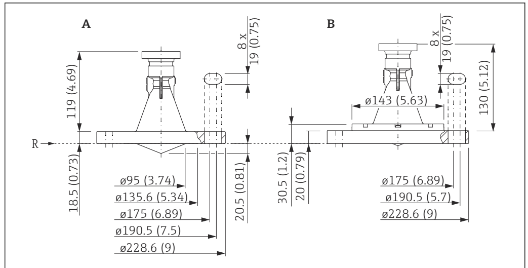
32 Dimensões do FMR56 com flange deslizante 4"/DN100. Unidade de medida mm (in)
