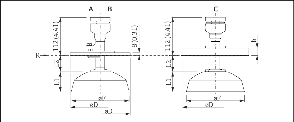
36 Dimensões do FMR57 com antena parabólica; unidade de engenharia: mm (pol.)
