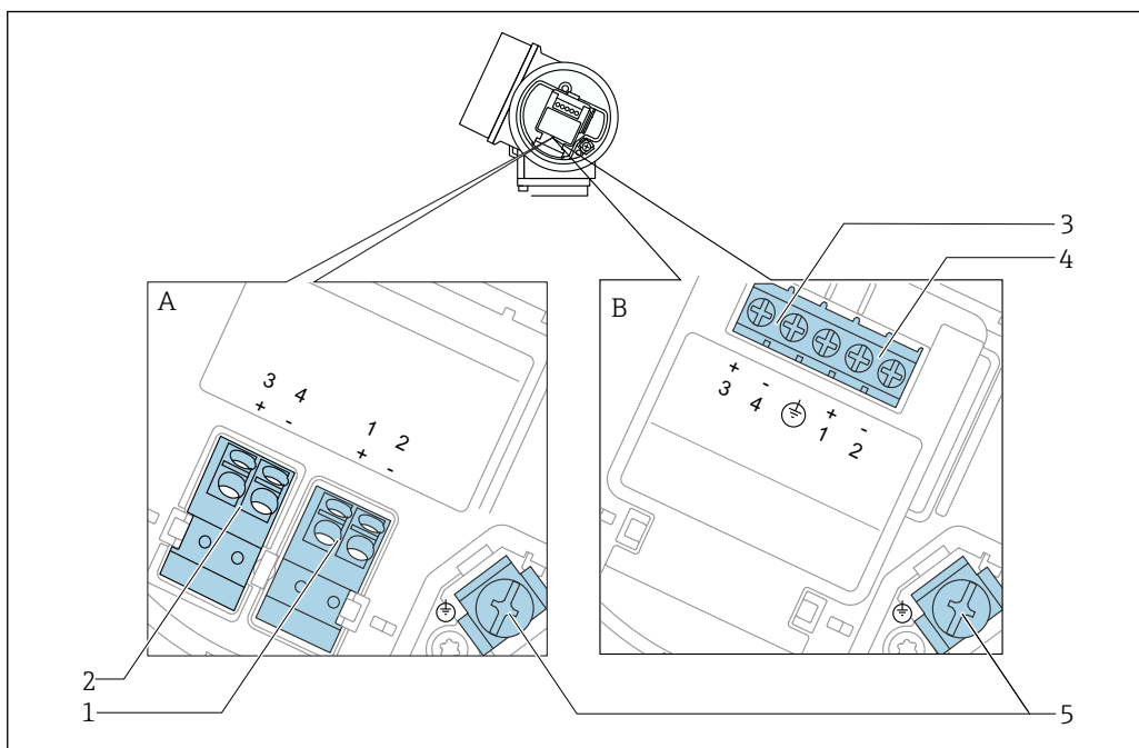
12 Esquema de ligação elétrica PROFIBUS PA / FOUNDATION Fieldbus
