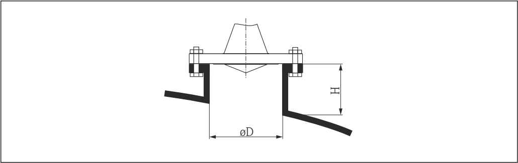
20 Diâmetro e altura do bocal para antenas piramidais com flange de deslizamento
