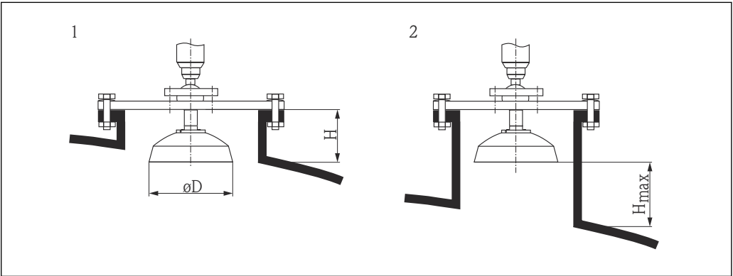
23 Montagem do bocal do Micropilot FMR57 com antena parabólica
