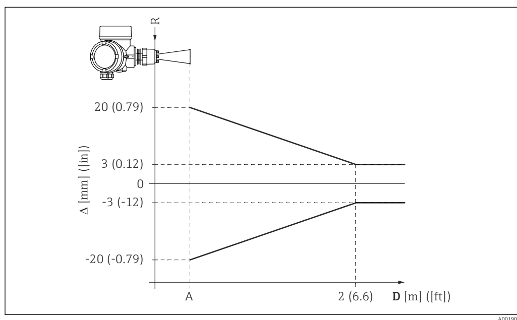
18 Erro máximo medido em aplicações de curto alcance
