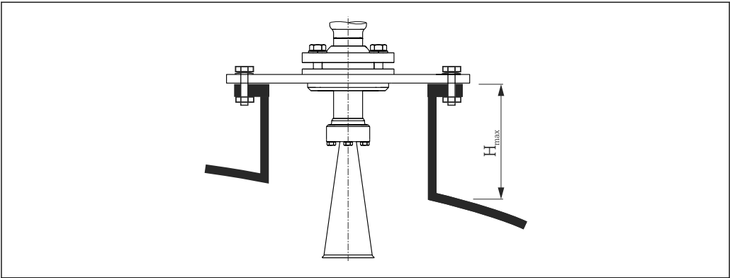
22 Altura do bocal para a antena piramidal (FMR57)
