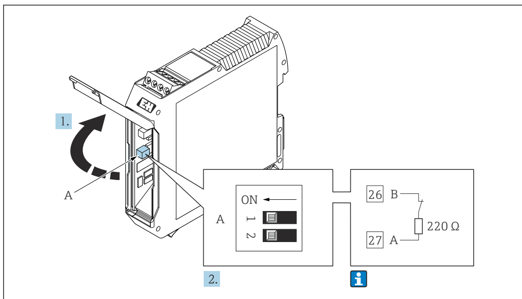
16 O resistor de terminação pode ser habilitado através da minisseletora na barreira de Promass 100
