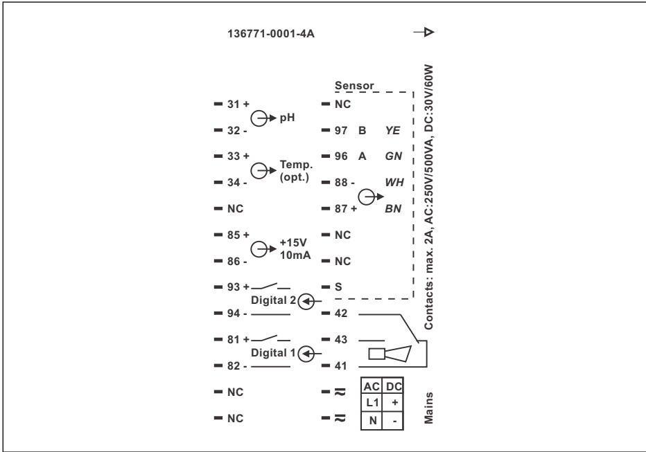
4 Etichetta connessioni/assegnazione dei morsetti
