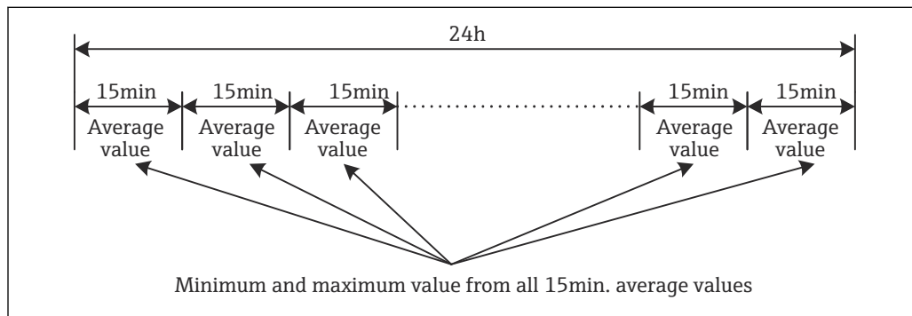
1 Registrering av de högsta och lägsta värdena på en dag (x = 15 min.)
