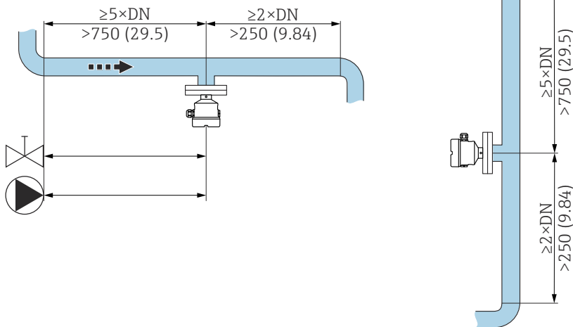
8 A bemeneti csőszakasz beépítése. Mértékegység mm (in)
