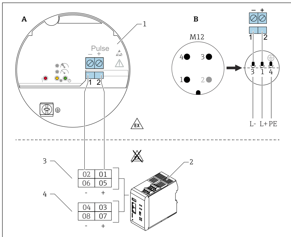
19 Csatlakozási rajz: a FEL60D elektronikus betét csatlakoztatása a QML51 sűrűségkalkulátorhoz
