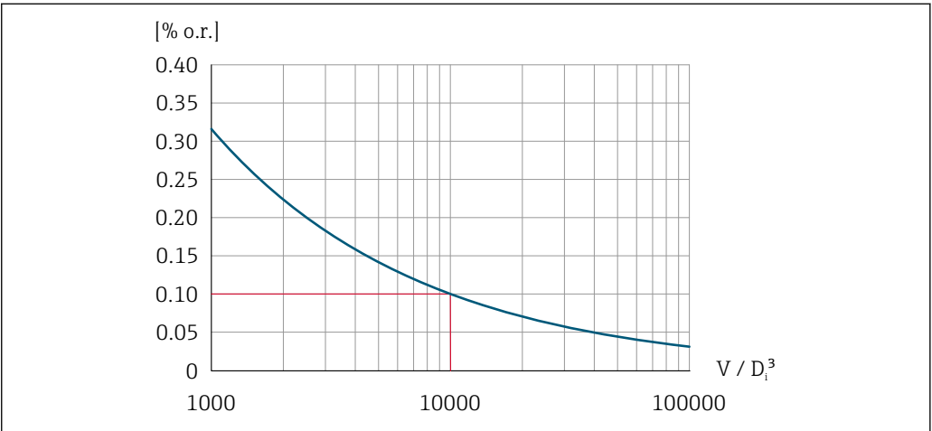
22 Reproductibilité = 0,1 % de m. avec un volume mesuré [m³] de V = 10000 \cdot D_i^3
