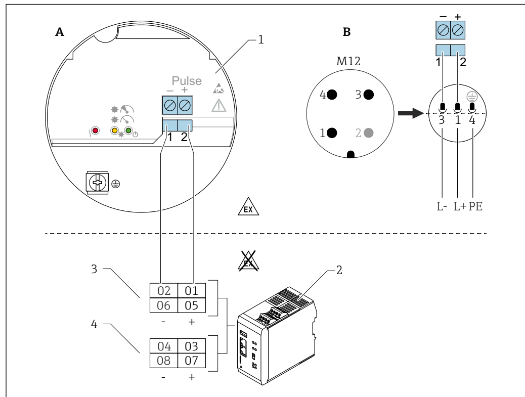
19 Anschlussschema: Anschluss Elektronikmodul FEL60D an den Dichterechner QML51
