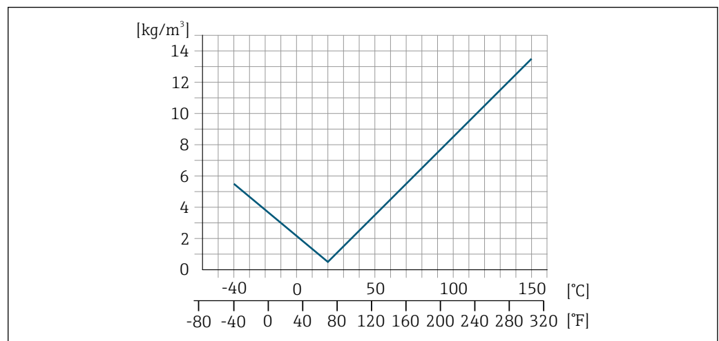
37 Ajustage sur site de la masse volumique, par exemple à +20 °C (+68 °F)
