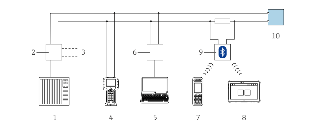
図 13 HART プロトコル経由のリモート操作オプション（パッシブ）
