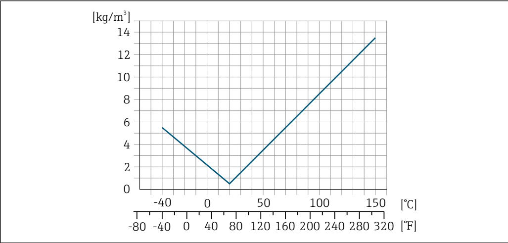
図 23 現場密度調整、例：+20 °C (+68 °F) 時
