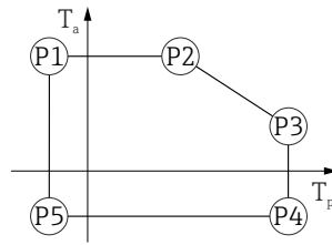
27 Caja de plástico; temperatura de proceso -20 \dots +200 \text{ }^{\circ}\text{C} ( -4 \dots +392 \text{ }^{\circ}\text{F} )
