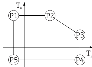
50 Caja de 316L, higiene; temperatura de proceso -20 ... +200 °C (-4 ... +392 °F)
