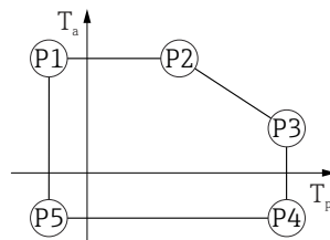
45 Caja de 316L; temperatura de proceso -40 ... +80 °C (-40 ... +176 °F)
