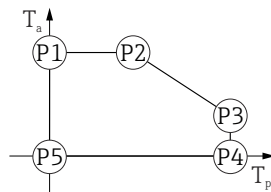
28 Caja de plástico; temperatura de proceso 0 \dots +200 \text{ }^{\circ}\text{C} ( +32 \dots +392 \text{ }^{\circ}\text{F} ) con homologación CSA C/US
