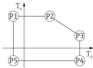
52 Caja de 316L, higiene; temperatura de proceso -40 ... +130 °C (-40 ... +266 °F)
