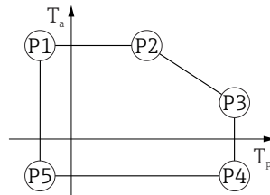
38 Caja de aluminio, recubierta; temperatura de proceso -20 \dots +200 \text{ }^{\circ}\text{C} ( -4 \dots +392 \text{ }^{\circ}\text{F} )
