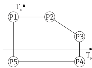
33 Caja de plástico; temperatura de proceso -40 \dots +150 \text{ °C} ( -40 \dots +302 \text{ °F} )
