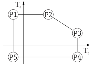
37 Caja de aluminio, recubierta; temperatura de proceso -20 \dots +150 \text{ }^{\circ}\text{C} ( -4 \dots +302 \text{ }^{\circ}\text{F} )
