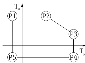
31 Caja de plástico; temperatura de proceso -40 \dots +130 \text{ °C} ( -40 \dots +266 \text{ °F} )
