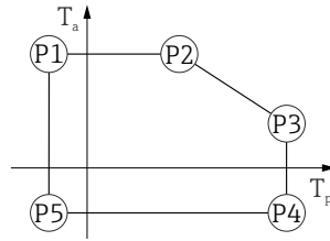
49 Caja de 316L, higiene; temperatura de proceso -20 ... +150 °C (-4 ... +302 °F)
