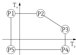
53 Caja de 316L, higiene; rango de temperatura de proceso: -40 ... +150 °C (-40 ... +302 °F)
