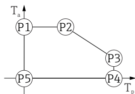
32 Caja de plástico; temperatura de proceso 0 \dots +130 \text{ °C} ( +32 \dots +266 \text{ °F} ) con homologación CSA C/US
