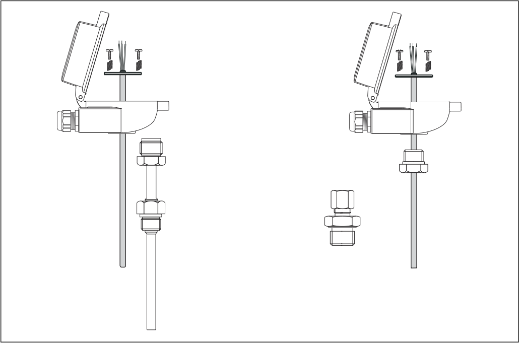
图 9 常规安装方式：安装在带保护套管的温度计中（左图）、直接接液测量（右图）
