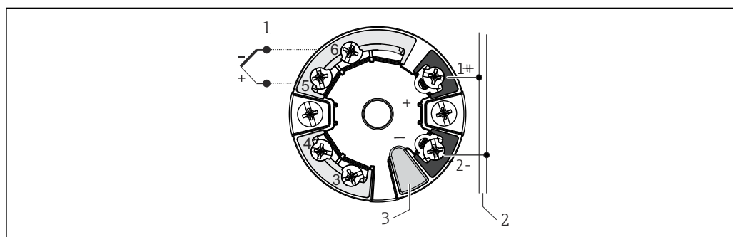
图 6 模块化变送器 iTEMP MT7x（单路传感器输入）
