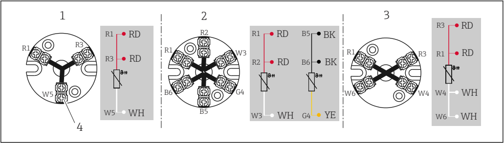
1 安装的陶瓷端子接线块
