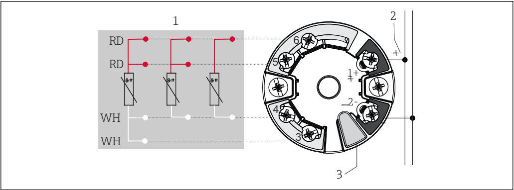
2 iTempt TMT7x 或 iTempt MT31 模块化变送器 (单路传感器输入)
