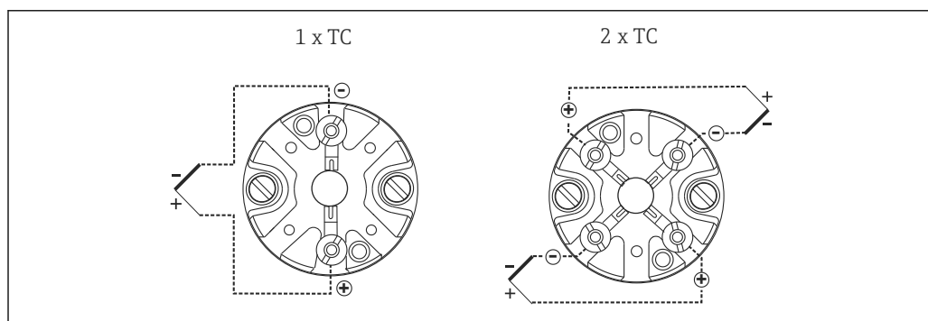
图 5 已安装陶瓷端子接线块
