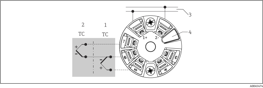
图 7 iTEMP TMT8x 模块化温度变送器（两路传感器输入）
