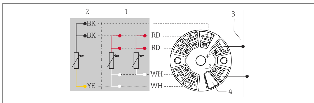
图 4 iTEMP TMT8x 模块化温度变送器（两路传感器输入）
