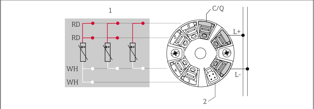
3 iTempt TMT36 模块化变送器 (单路传感器输入)
