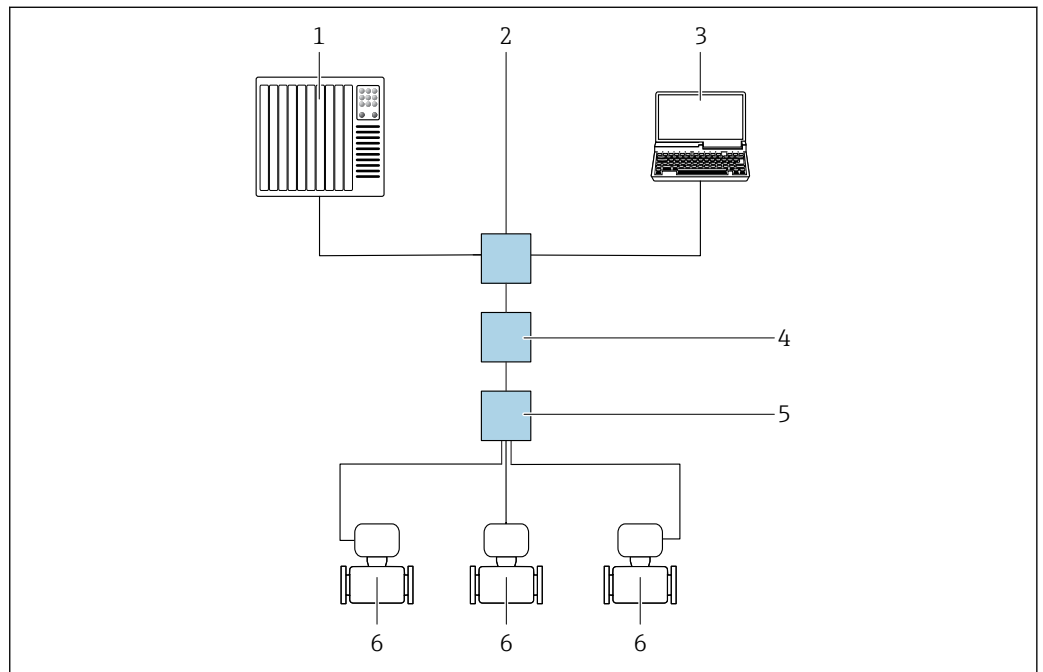
22 Opções para operação remota através do protocolo Modbus TCP por Ethernet-APL (ativa)
