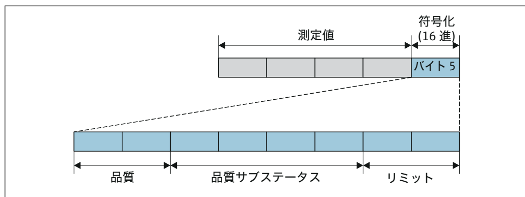
図 41 ステータスバイトの構造
