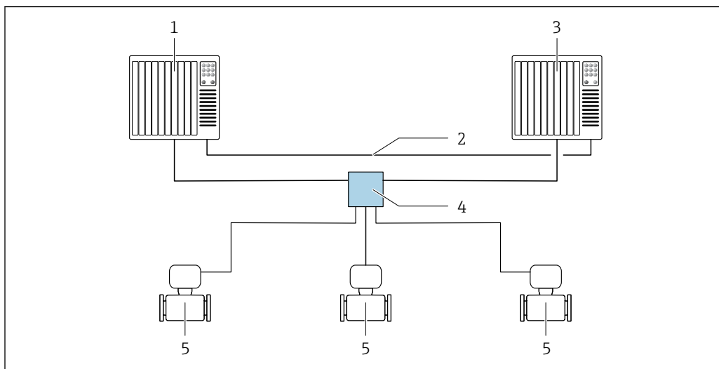
図 36 冗長システム (S2) のレイアウト例：スター型トポロジー
