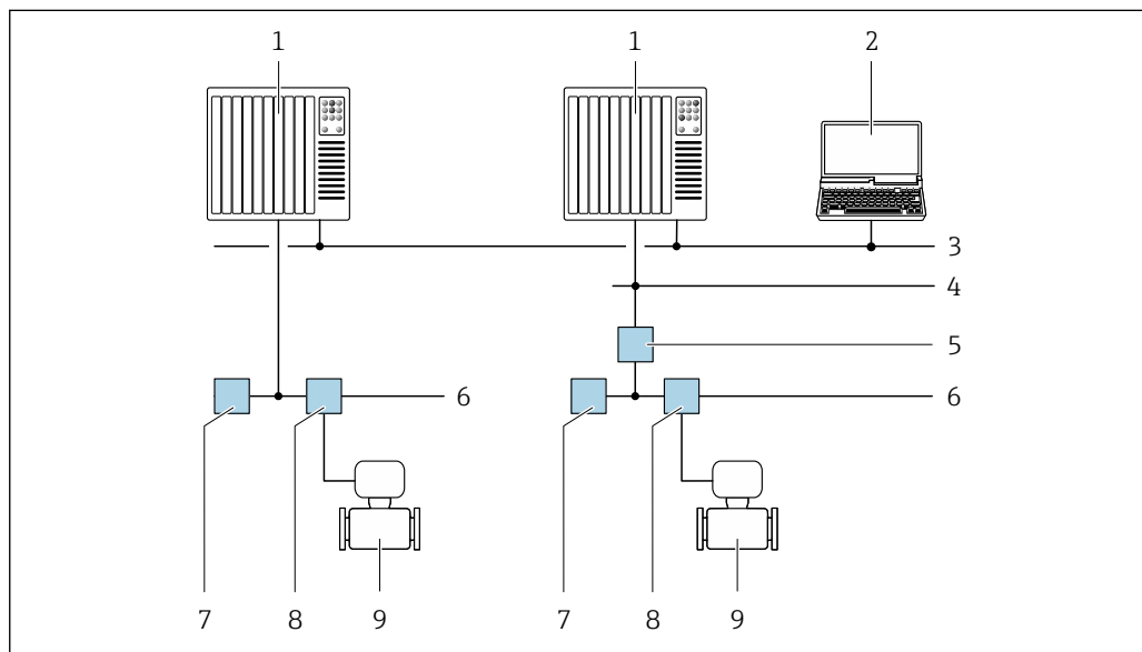
25 Варианты дистанционного управления по сети FOUNDATION Fieldbus
