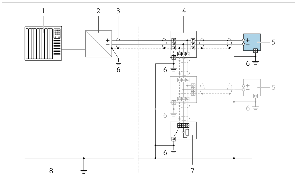
19 Пример подключения для интерфейса FOUNDATION Fieldbus
