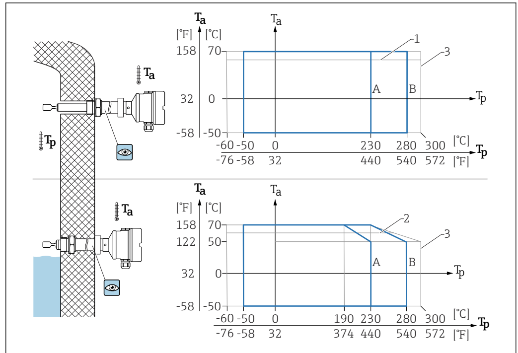
51 Zulässige Umgebungstemperatur T_a am Gehäuse in Abhängigkeit von der Prozesstemperatur T_p im Behälter
