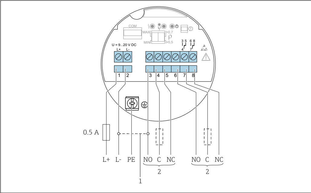
24 Gleichstromanschluss mit Relaisausgang, Elektronikeinsatz FEL64 DC 1 Im gebrückten Zustand arbeitet der Relaisausgang in Form einer NPN-Logik 2 Anschließbare Last
