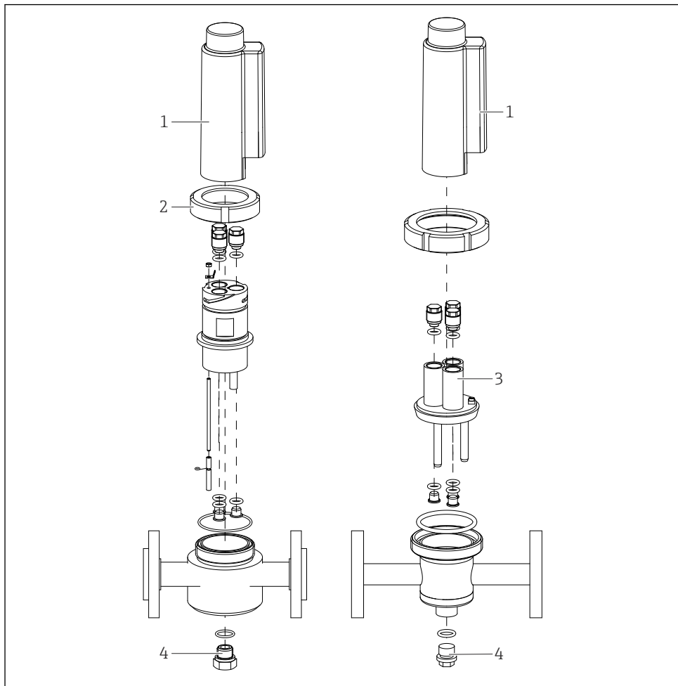
1 Aufbau CPA240-2xxxxxx (links) und CPA240-3xxxxxx (rechts)
