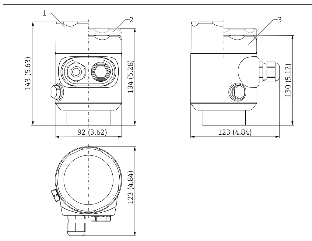
図 25 シングルコンパートメントハウジング、SUS 316L 相当、サニタリ仕様の寸法。測定単位 mm (in)
