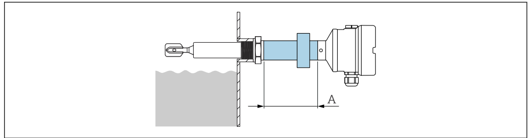
図 28 伸長パイプ用の耐圧防爆対応ガスタイトフィードスルー
