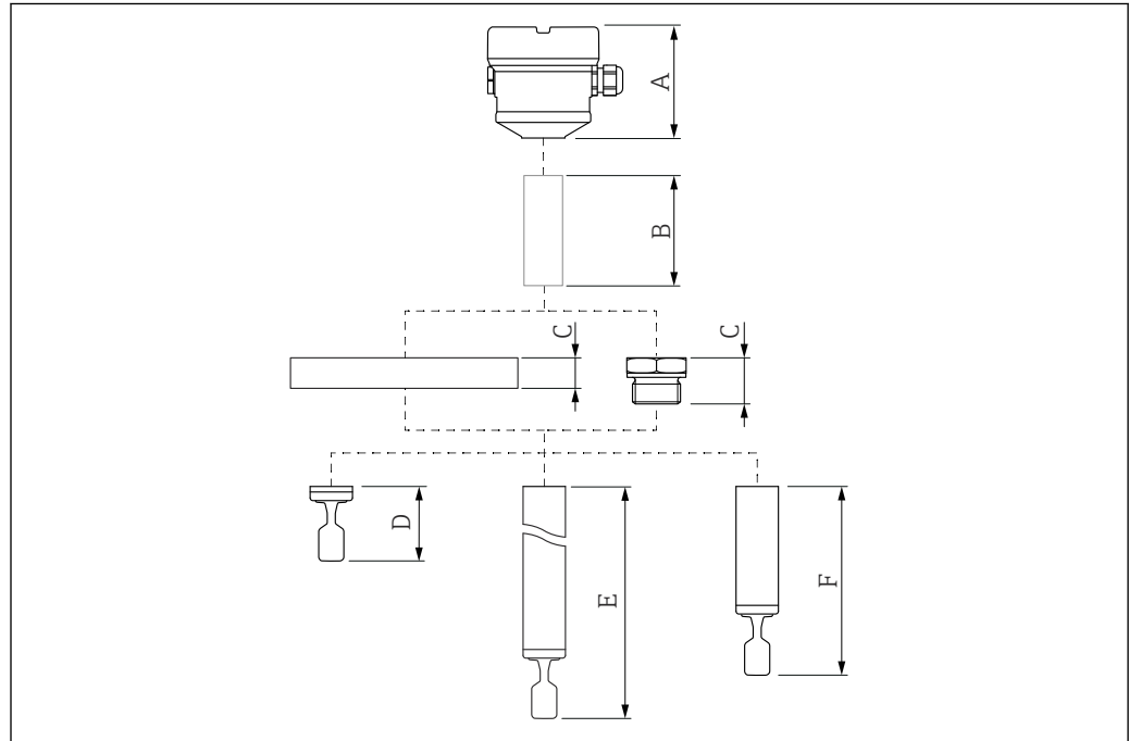
図 22 本体高さを計算するための構成品
