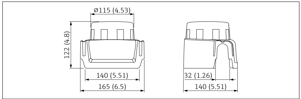
図 47 アルミニウム製シングルコンパートメントハウジング用保護カバー。測定単位 mm (in)
