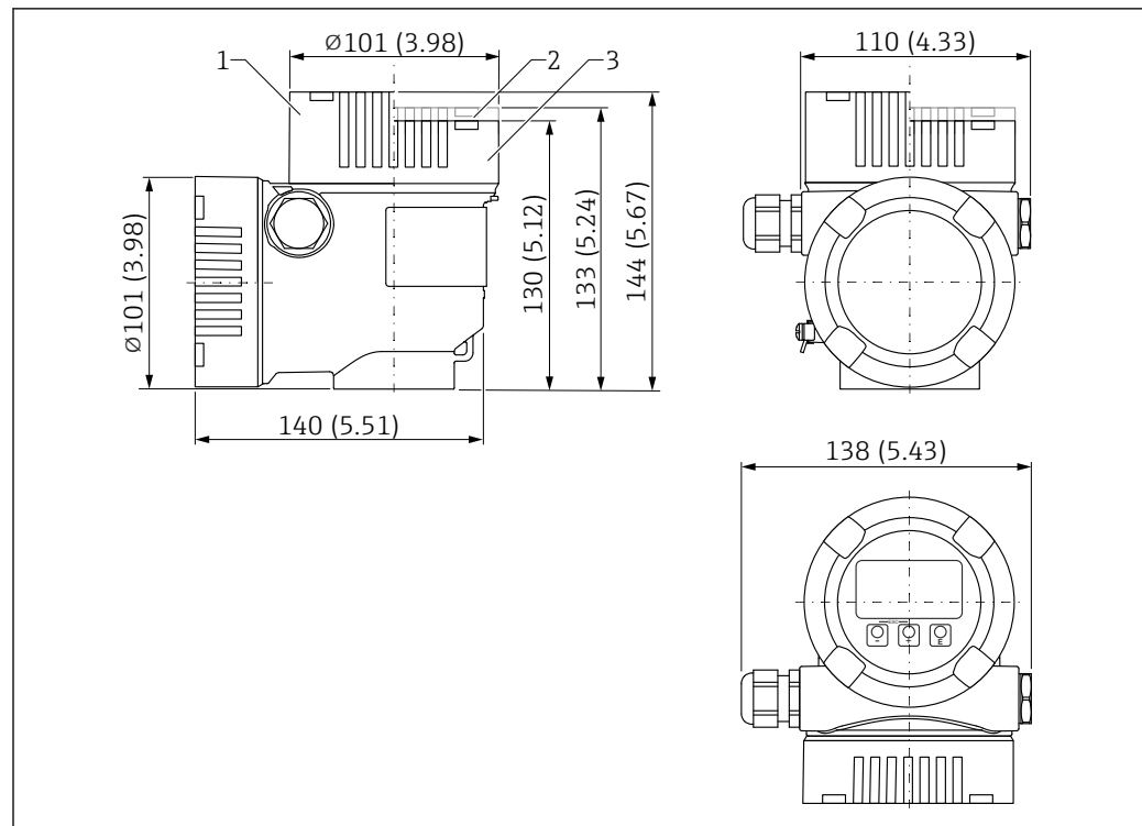
図 27 寸法；デュアルコンパートメントハウジング L 字型（SUS 316 L 相当）；M20 カップリングおよびプラグ（プラスチック）付き。測定単位 mm (in)
