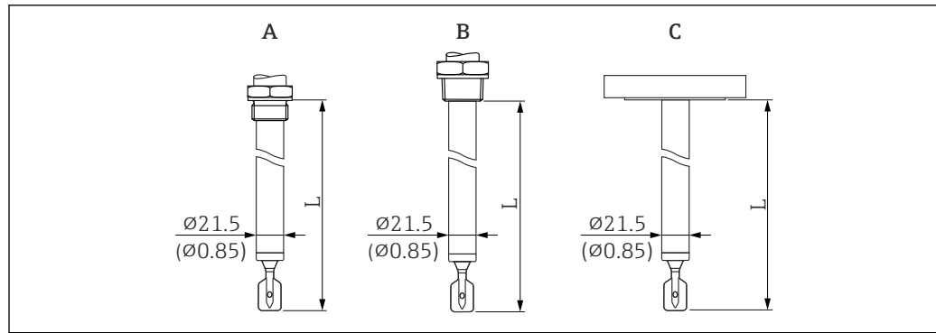
図 30 プローブ型式：伸長パイプ、ショートパイプ（センサ長 L）。測定単位 mm (in)
