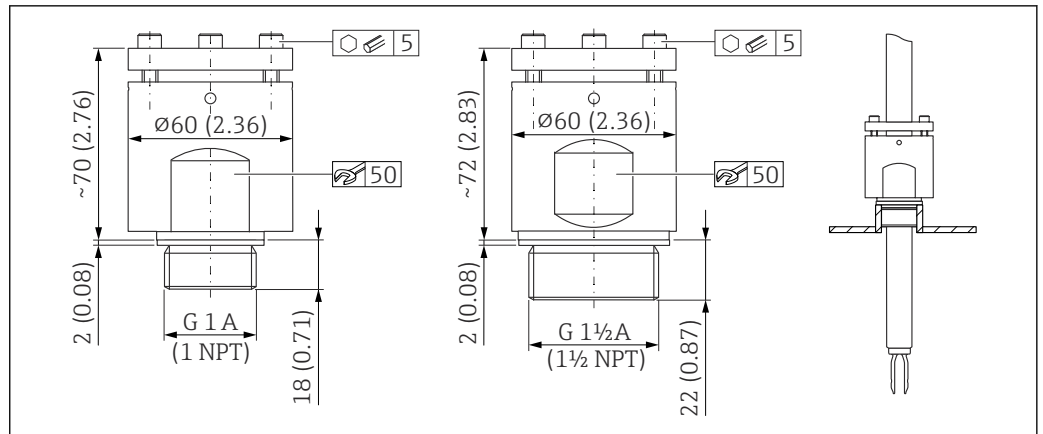
図 50 高圧用スライディングスリーブ。測定単位 mm (in)
