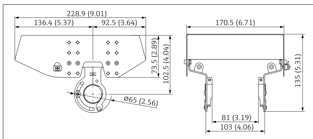
図 46 デュアルコンパートメントハウジング用の日除けカバー。測定単位 mm (in)
