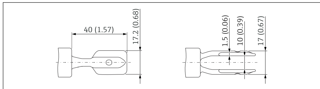
図 31 音叉部。測定単位 mm (in)
