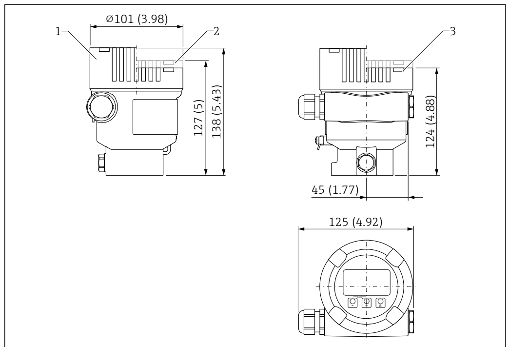
図 24 シングルコンパートメントハウジング、アルミニウム、コーティングの寸法。測定単位 mm (in)
