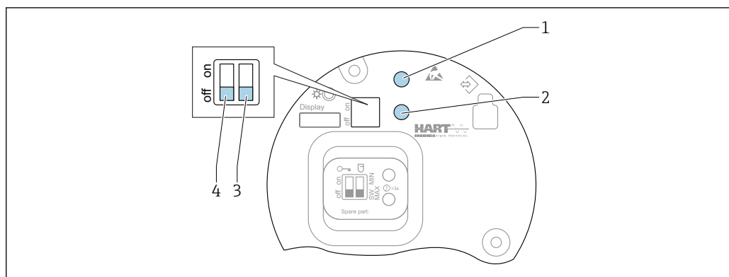
図 44 FEL60H エレクトロニックインサートの操作キーおよび DIP スイッチ
