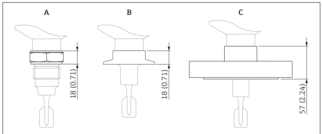
図 32 プロセス接続の最大高さ仕様。測定単位 mm (in)
