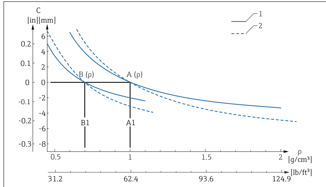
図 6 密度に対するスイッチポイント偏差
