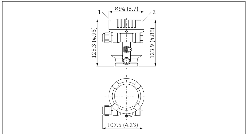
図 23 寸法；シングルコンパートメントハウジング（プラスチック）；M20 カップリングおよびプラグ（プラスチック）付き。測定単位 mm (in)
