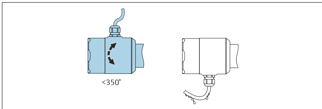
図 14 ロックネジのないドリッブループ付きハウジング
