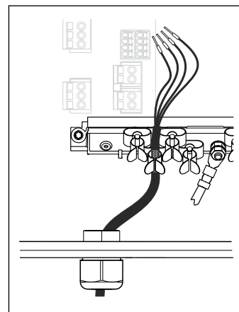
图 22 将电缆安装在接地夹中
