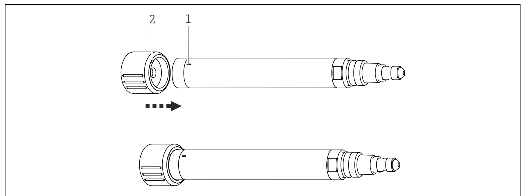
图 18 将固态标定模块安装在传感器上
