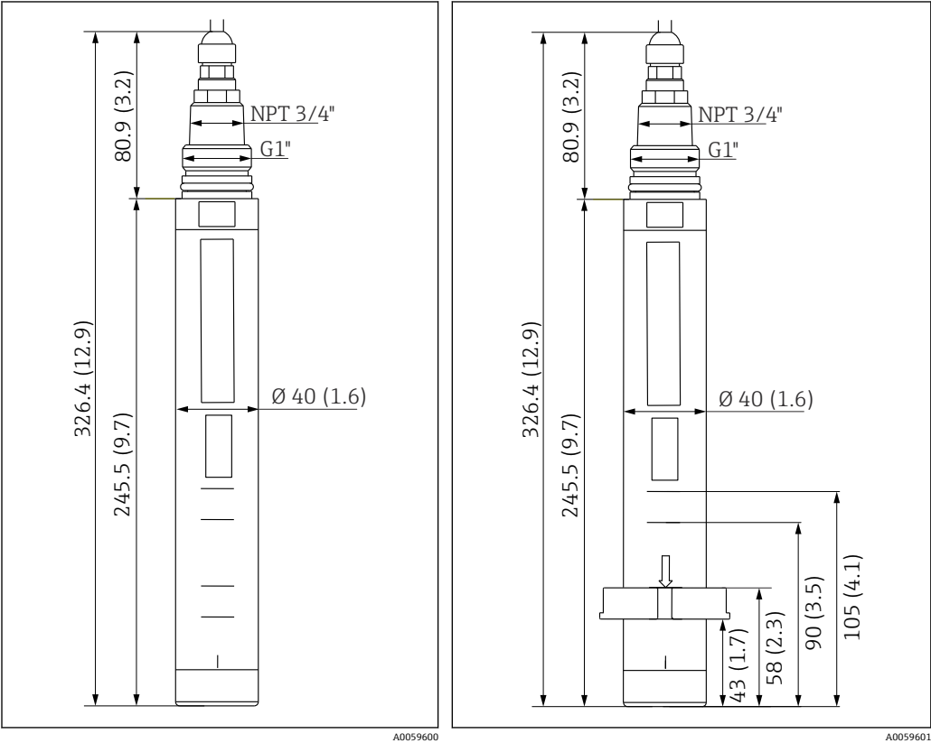
图 2 传感器的外形尺寸；单位：mm (in) 图 3 传感器（带卡环）的外形尺寸；单位：mm (in)
