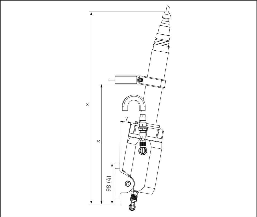
5 安装在 CFS51 标准安装支架中的传感器外形尺寸；单位：mm (in)
