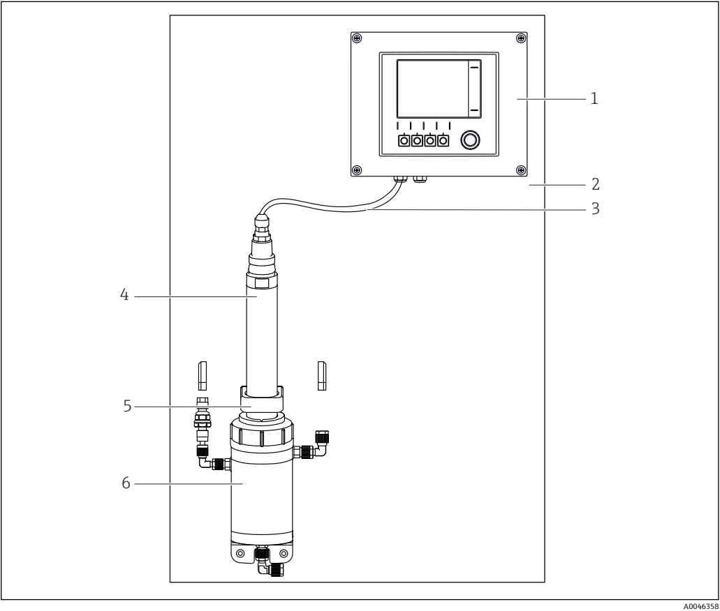
图 13 测量系统
