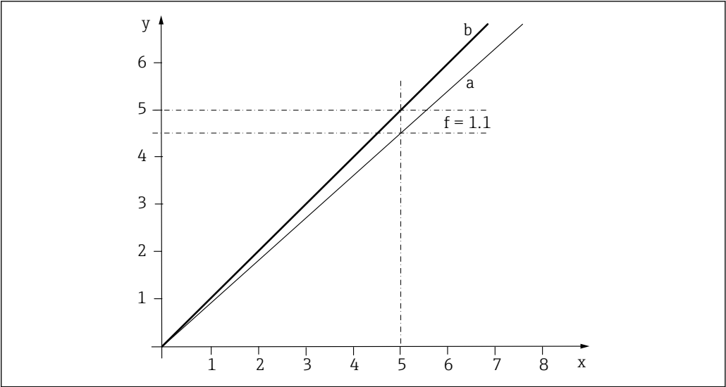
28 系数标定原理
