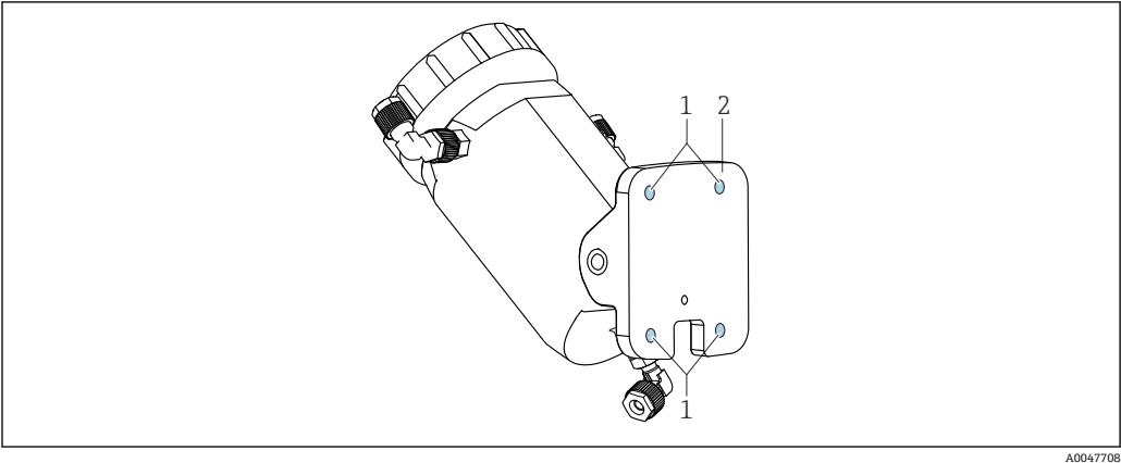
15 安装支架后视图 1 M5 螺丝 (非标准供货件) 安装孔 2 固定板
