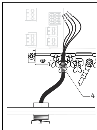
图 21 将电缆连接至接地夹
