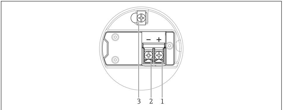
☞ 3 연결부의 연결 단자 및 접지 단자
