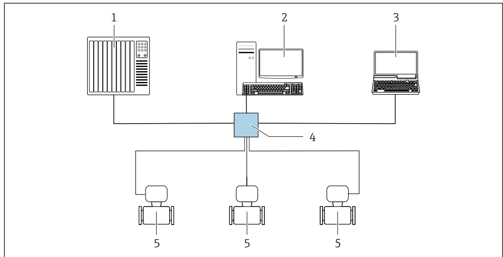
图 32 通过 EtherNet/IP 网络进行远程操作：星形拓扑结构
