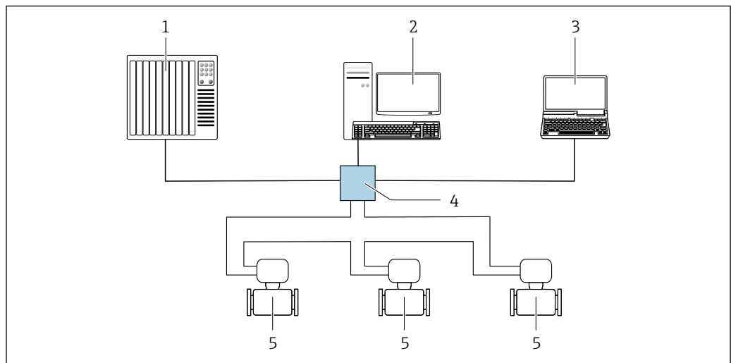
图 33 通过 EtherNet/IP 网络进行远程操作：环形拓扑结构
