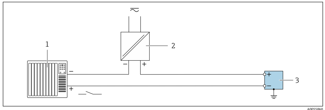
图 26 状态输入
