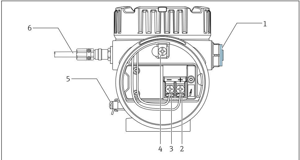
34 NMT81-klemme (ATEX · Ex ia)
